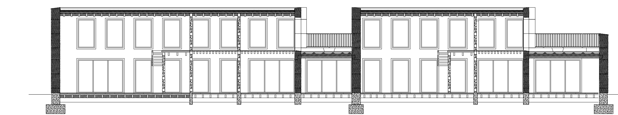
COUPE LONGITUDINALE
