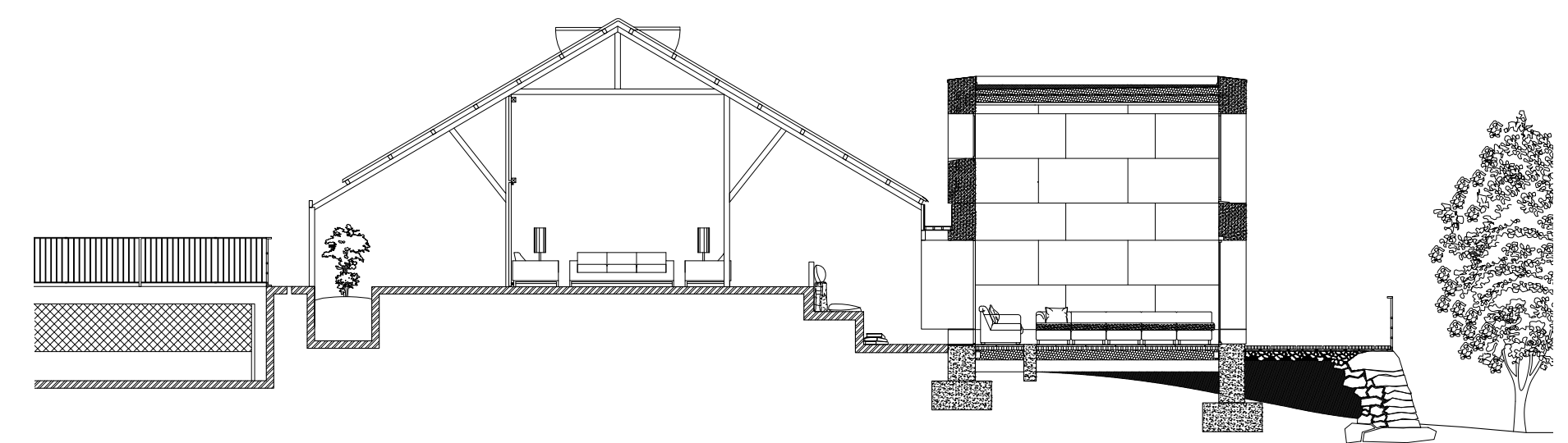
COUPE "SALON"
