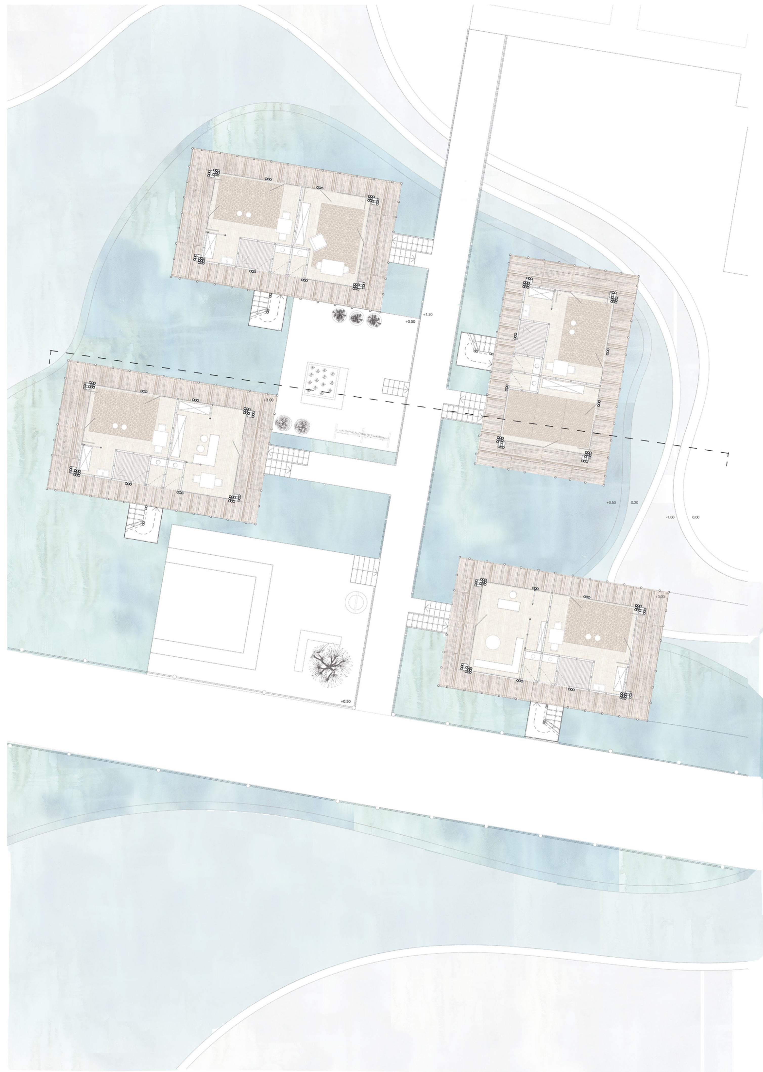
Plan/Plan masse 1/25
