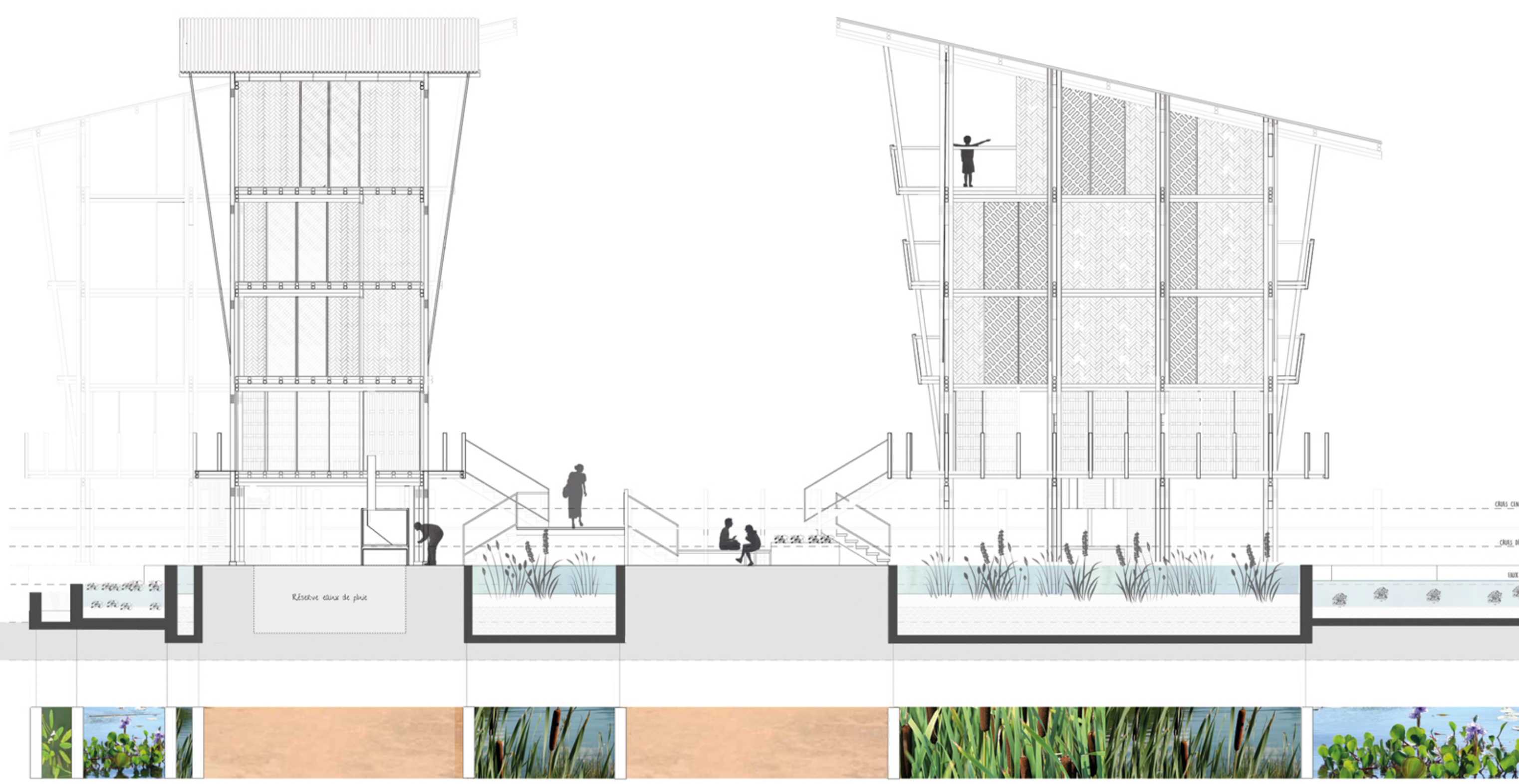
Coupe/Façade 1/100
