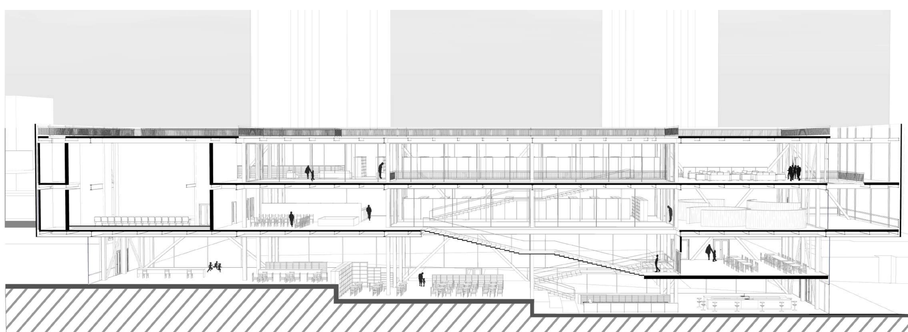
Coupe perspective 1/200 ème
