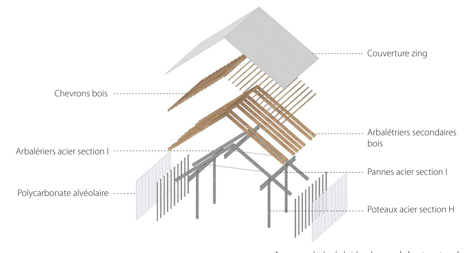
Axonomie éclatée du module structurel
