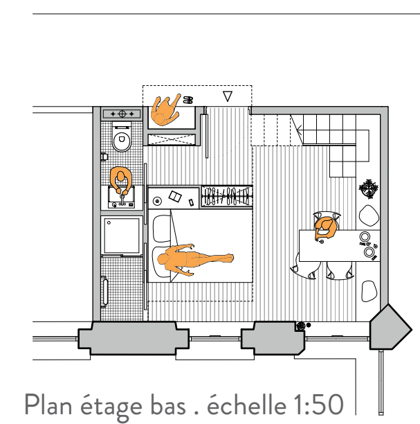
Plan étage bas . échelle 1:50
