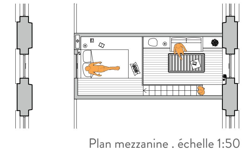
Plan mezzanine . échelle 1:50
