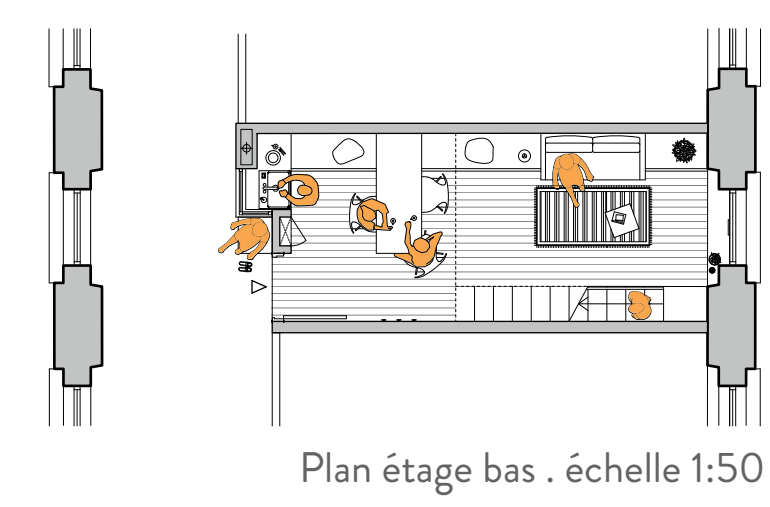
Plan étage bas . échelle 1:50
