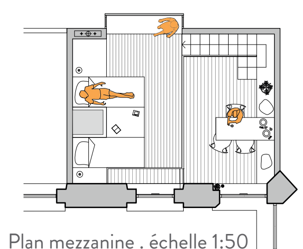
Plan mezzanine . échelle 1:50
