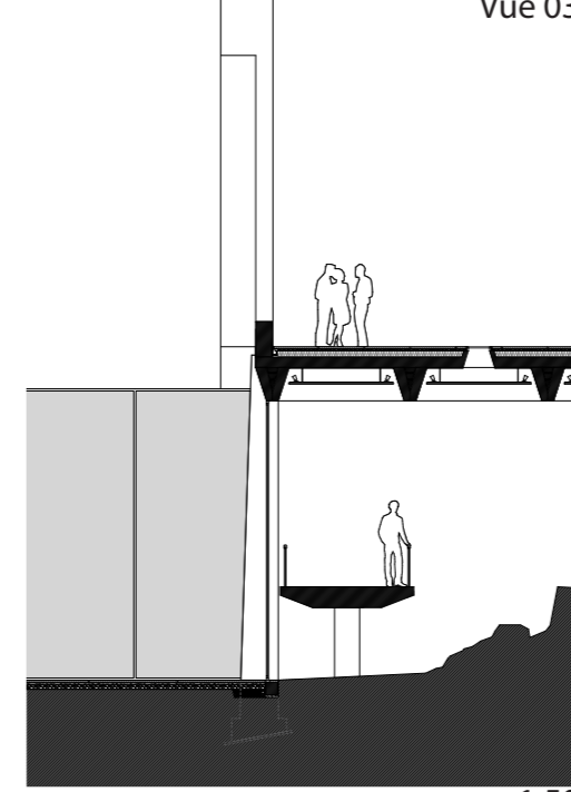
coupe1:50
