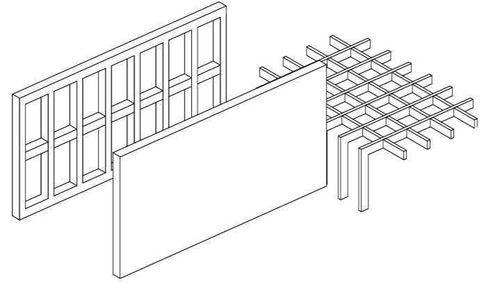
Poutres voiles / plafond à caisson
