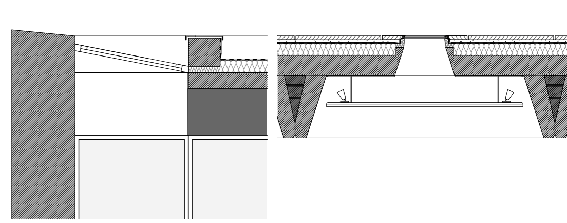
Détail 1:20
