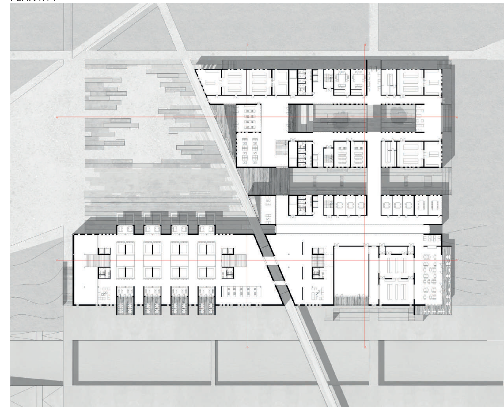
PLAN REZ-DE-CHAUSSEE
