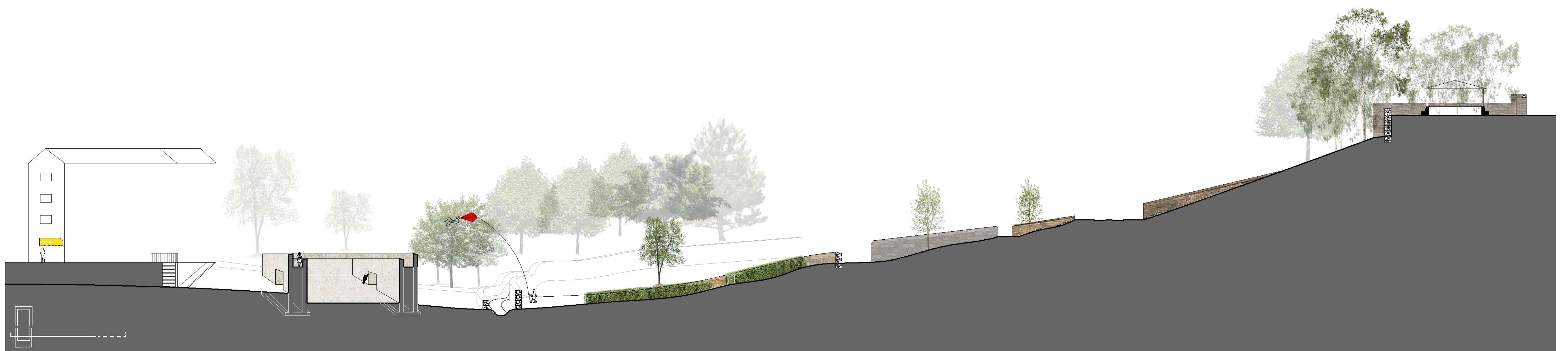
THEATRE EN PLEIN AIR, COUPE PAYSAGERE TRANSVERSALE, 1.250e, DOUBLE PENTE, RAPPORT A L'EAU ET AUX DEUX TERRASSES, SEULES HORIZONTALES DU PARC
