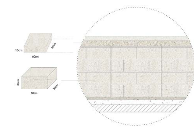
COUPE DETAIL, THEATRE EN PLEIN AIR, 1.50e
