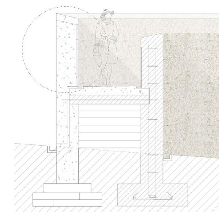
COUPE DETAIL, THEATRE EN PLEIN AIR, 1.50e
