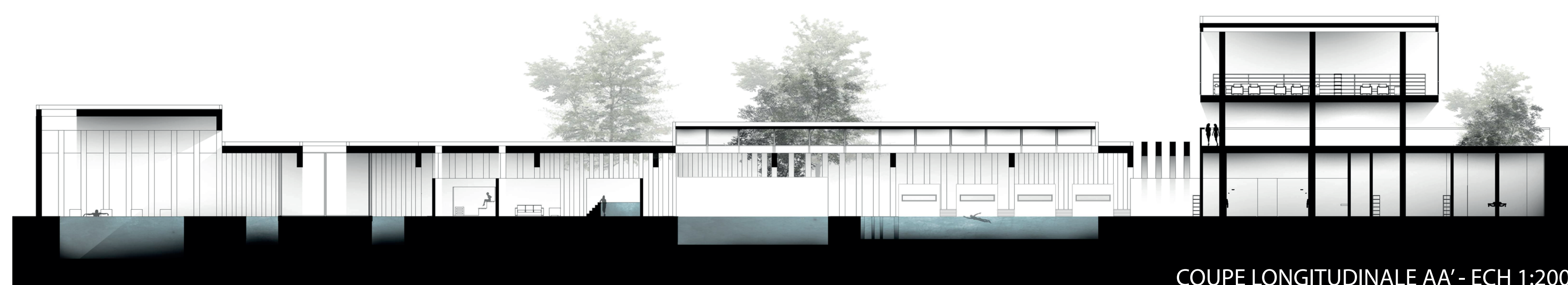
COUPE LONGITUDINALE AA' - ECH 1:200
