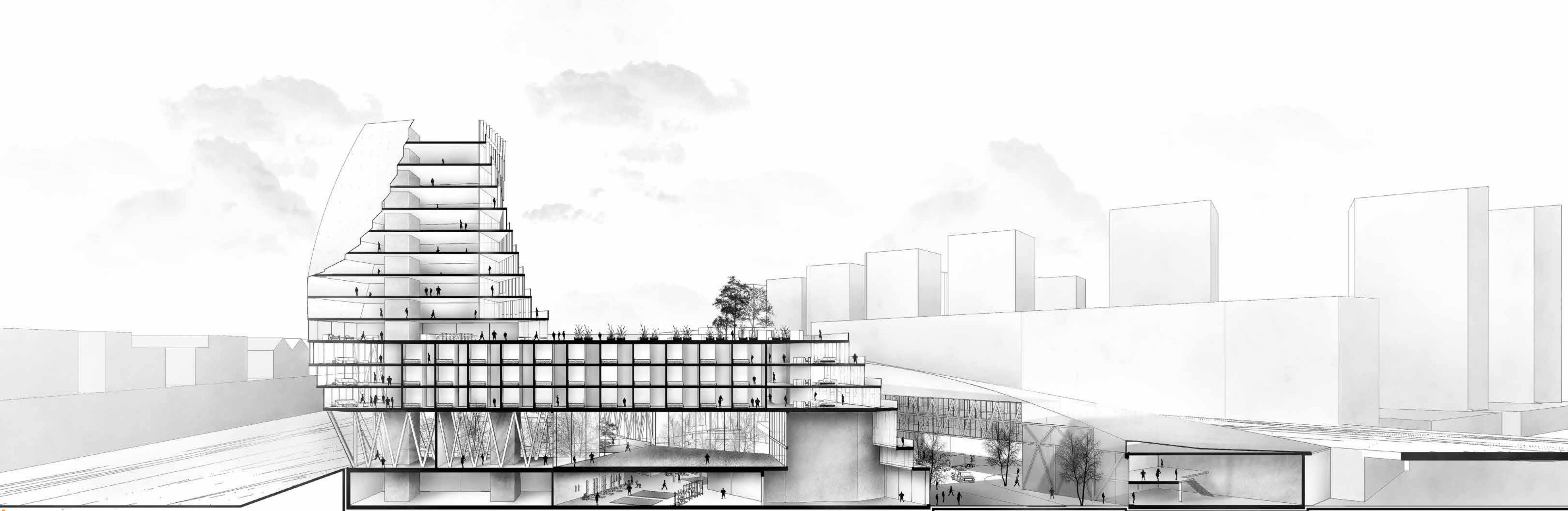
Coupe sur la Tour 1:200
