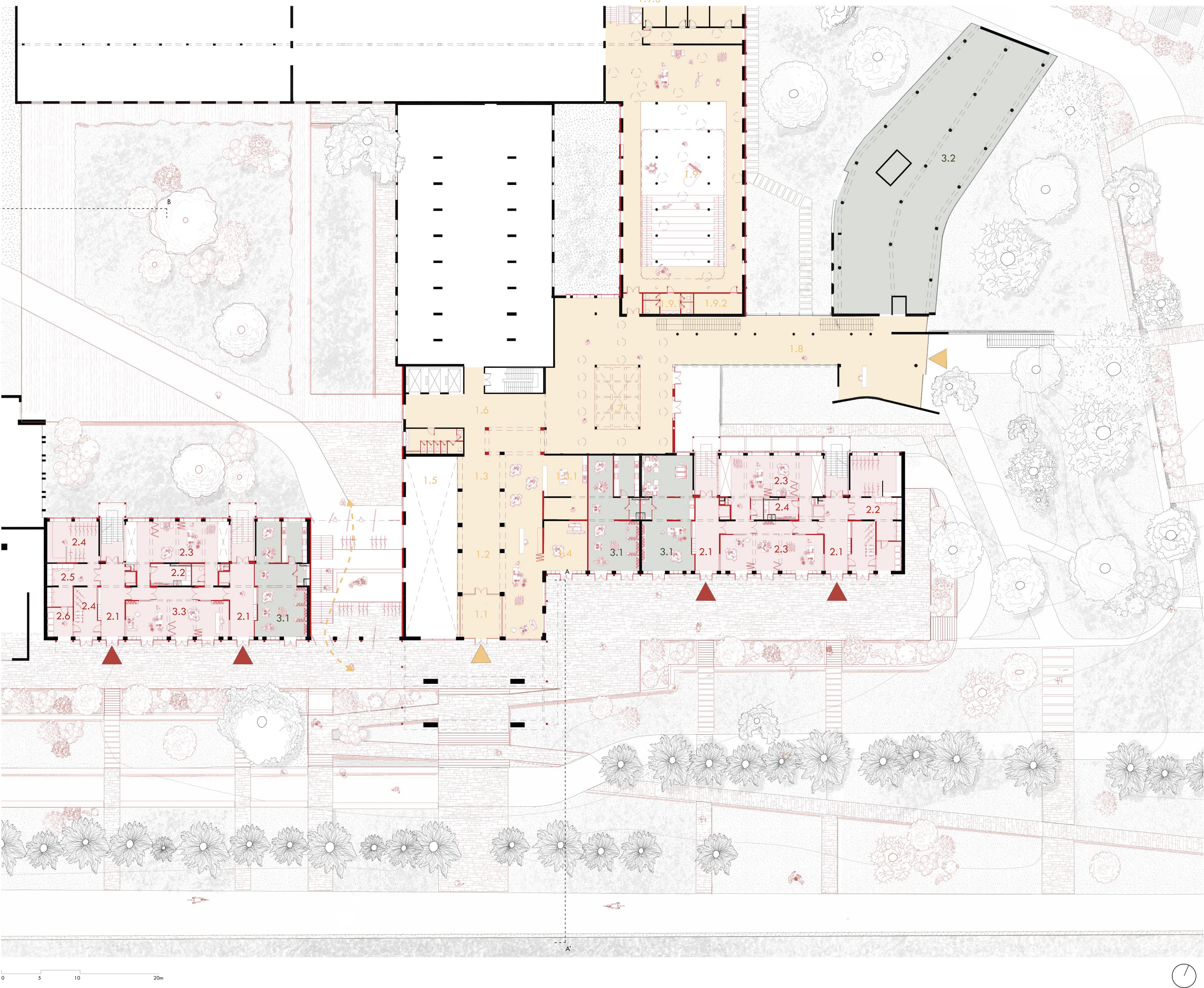
PLAN DE REZ-DE-CHAUSSÉE - 1/200
