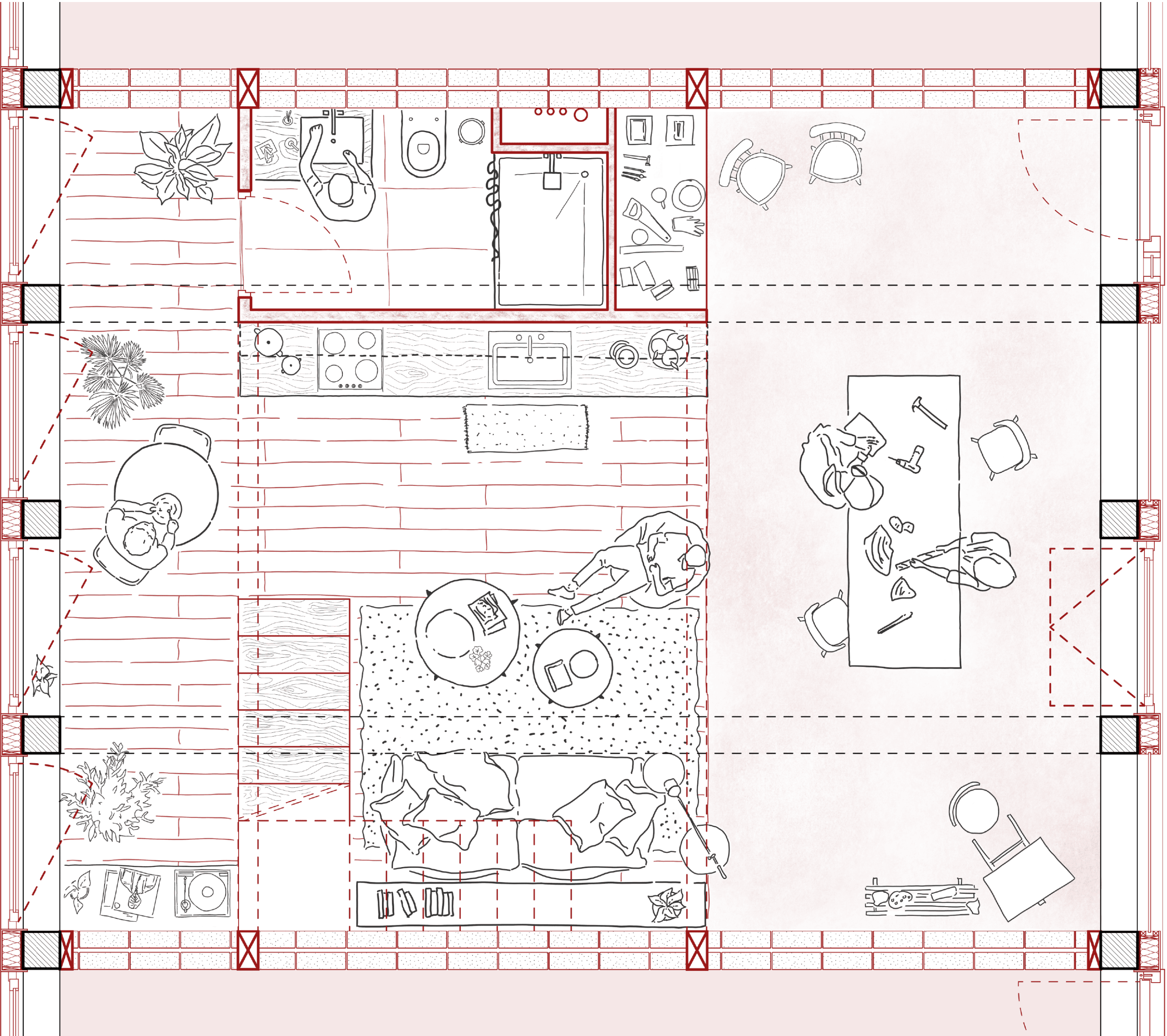
Plan Atelier-Logement 1/20
