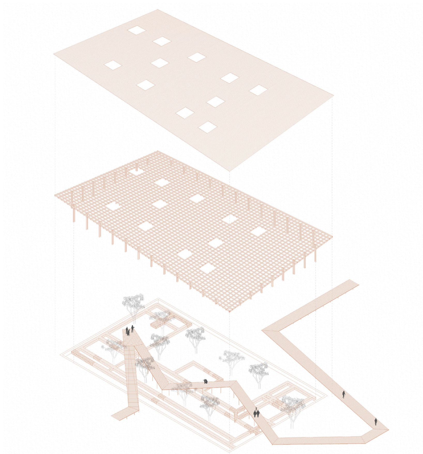
REVELER LES VESTIGES_PAVILLON ARCHEOLOGIQUE
