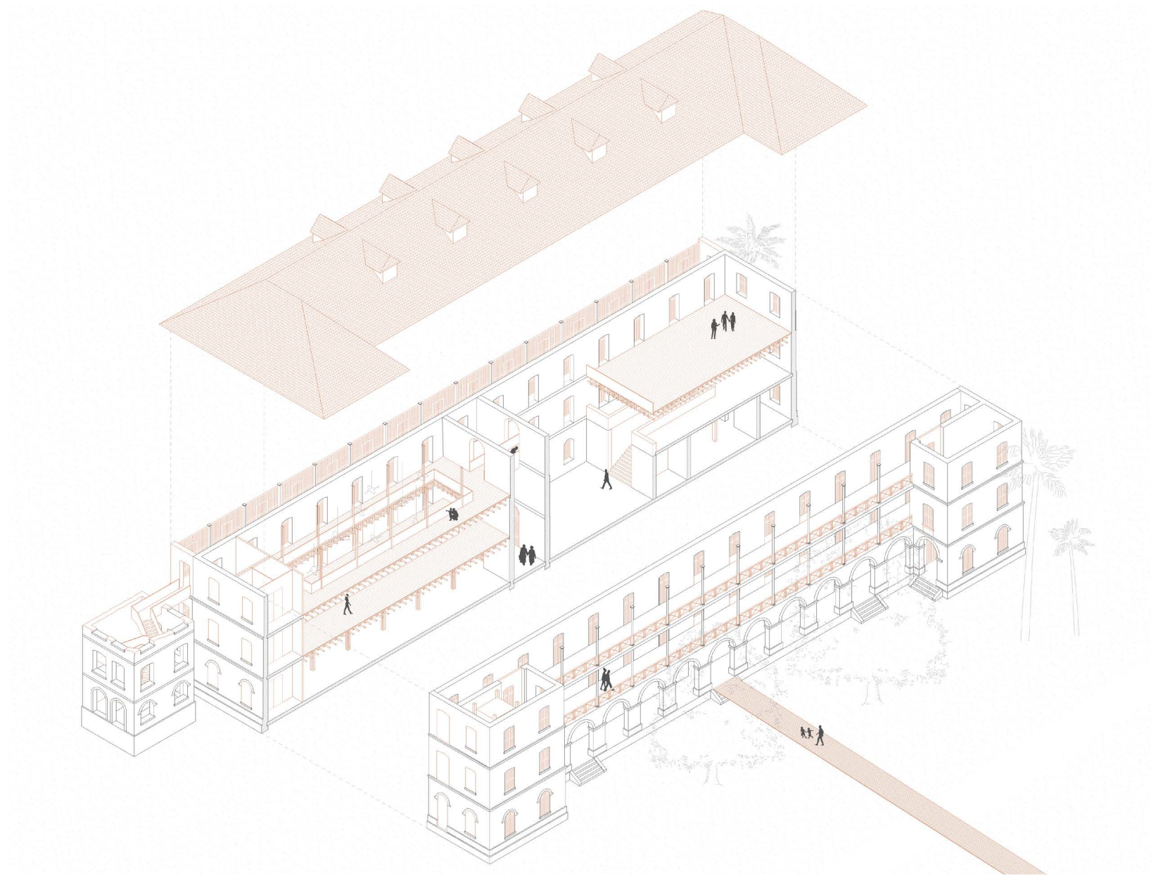
SOUVENIR ET DECOUVERTE_BATIMENT D'EXPOSITION
