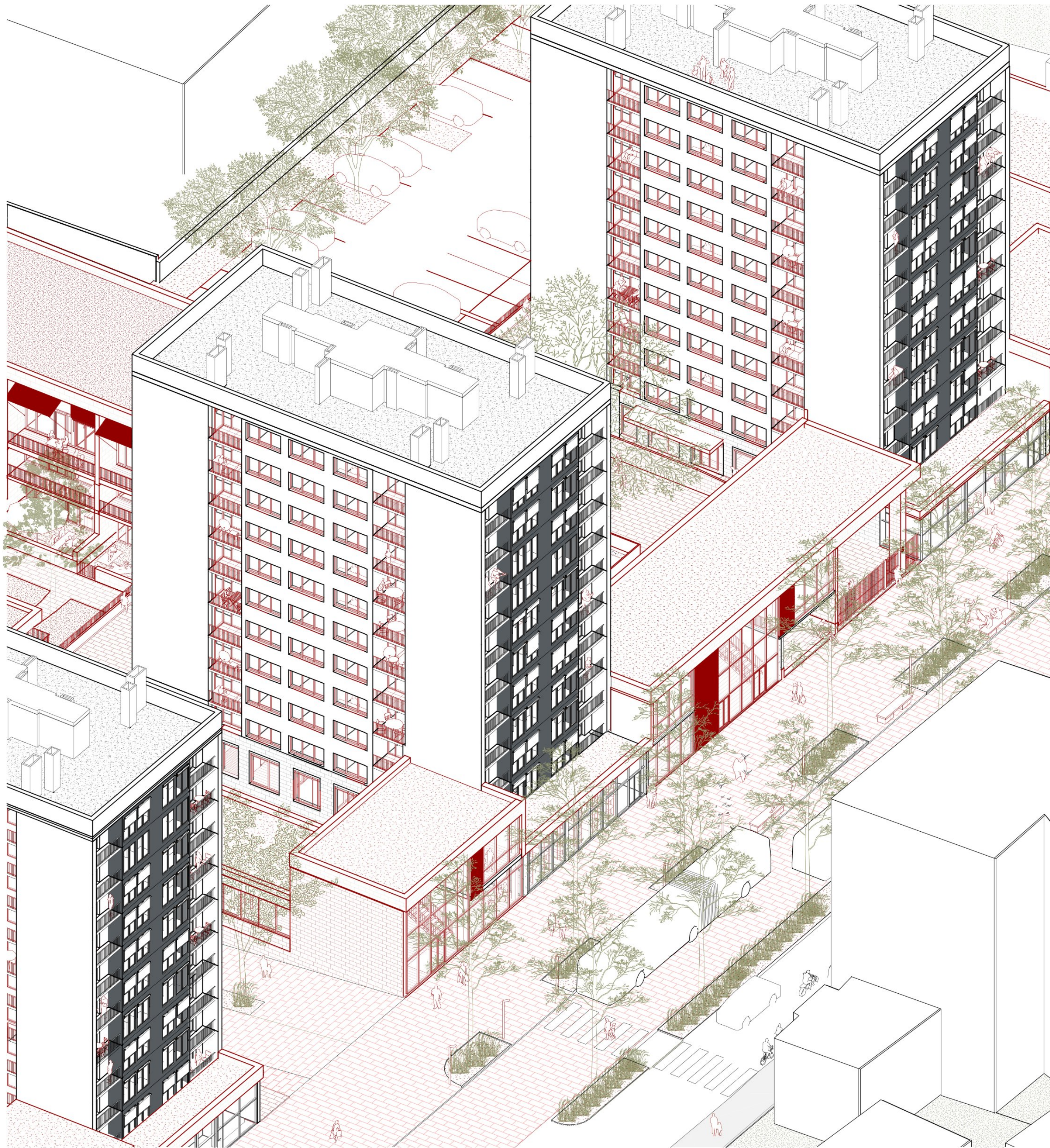
AXONOMÉTRIE : DU REZ-DE-VILLE AU REZ DE JARDIN - 1 : 200
