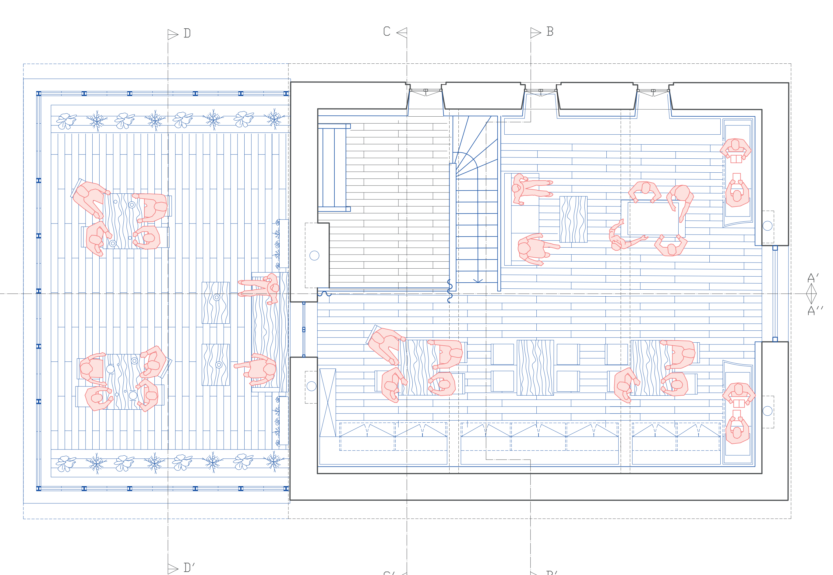
Plan R+2 Echelle : 1/50
