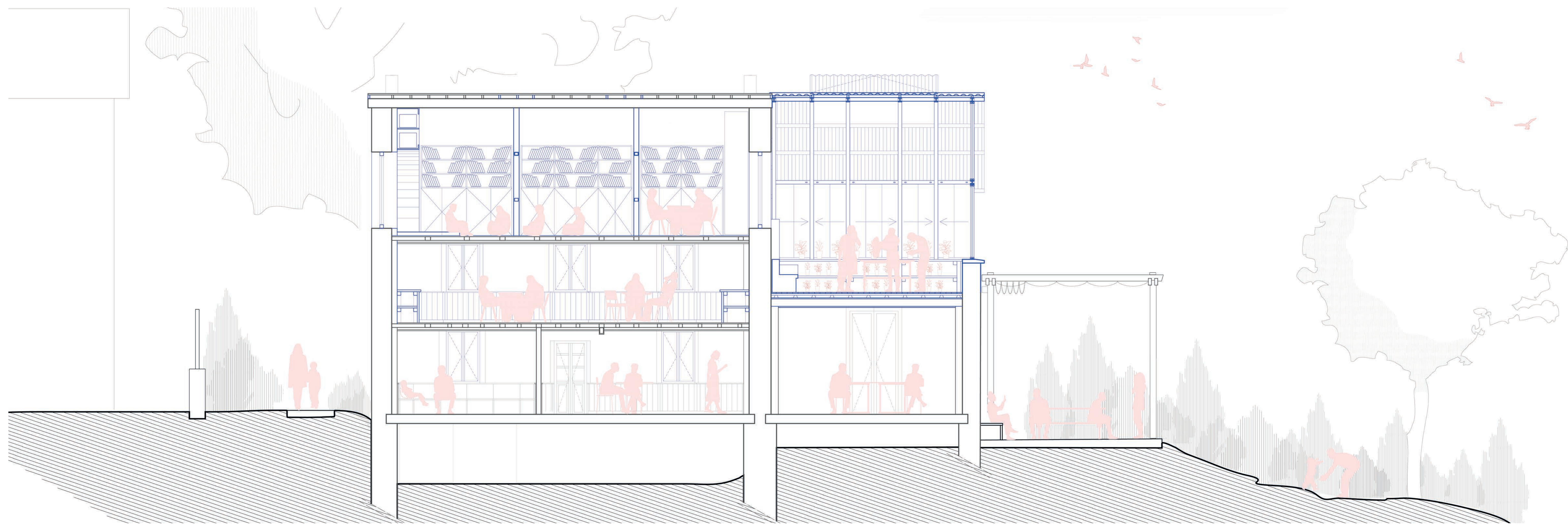
Coupe A-A'' Echelle : 1/50
