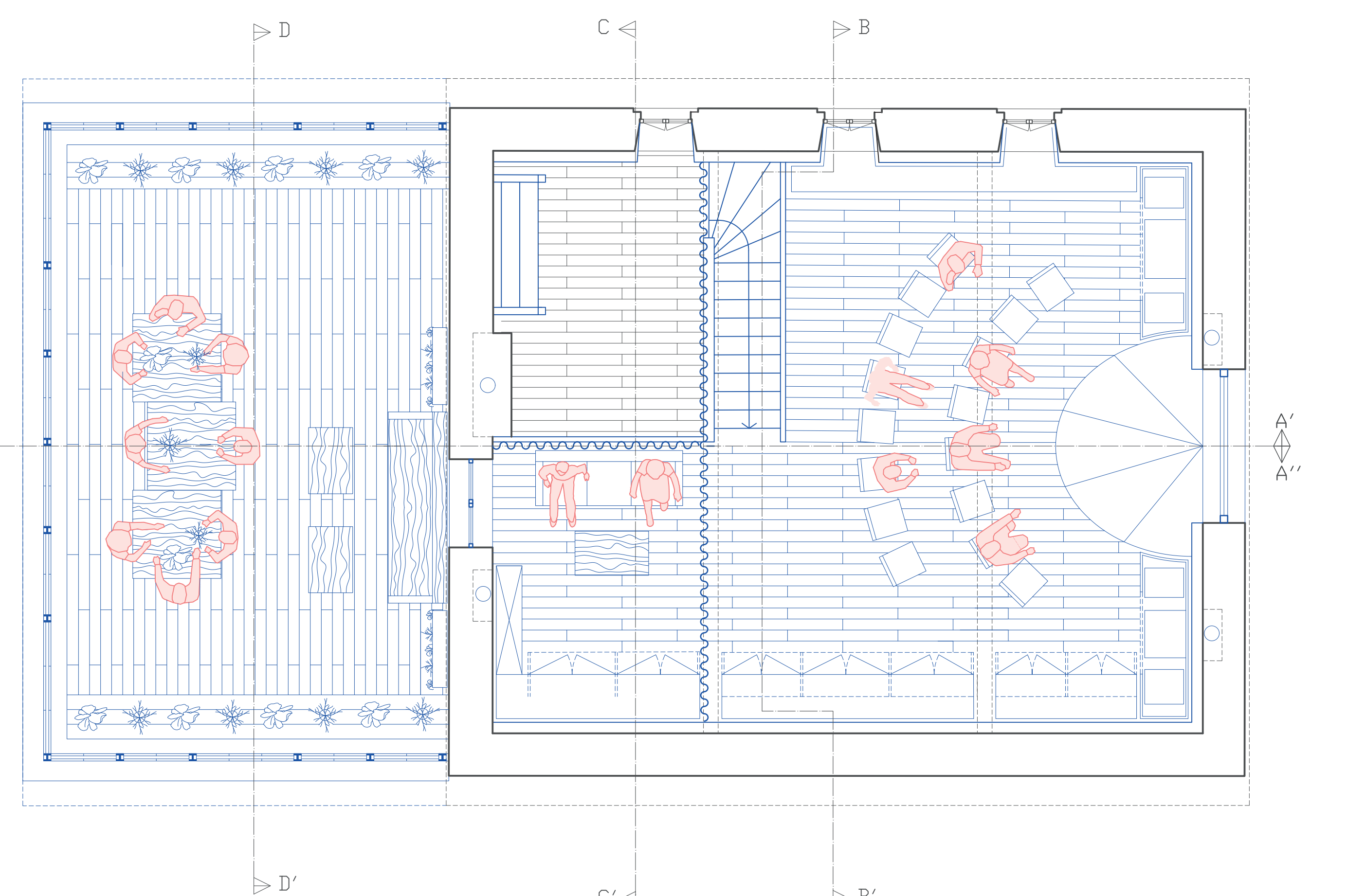
Plan R+2 Echelle : 1/50
