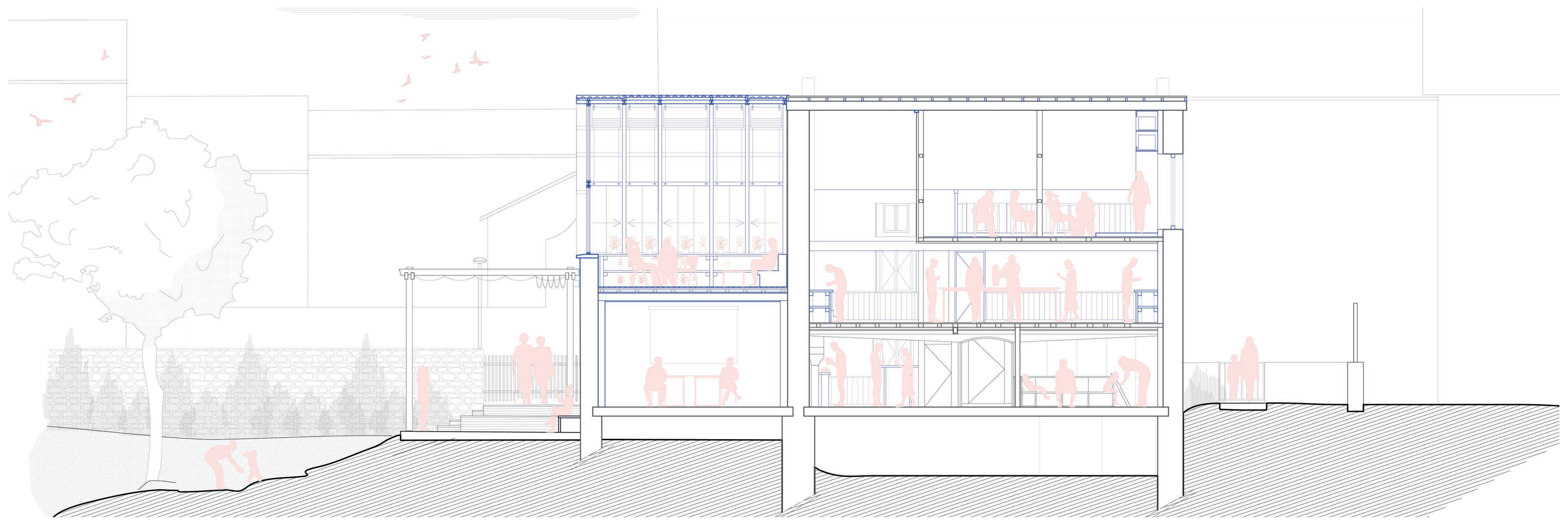
Coupe A-A' Echelle : 1/50
