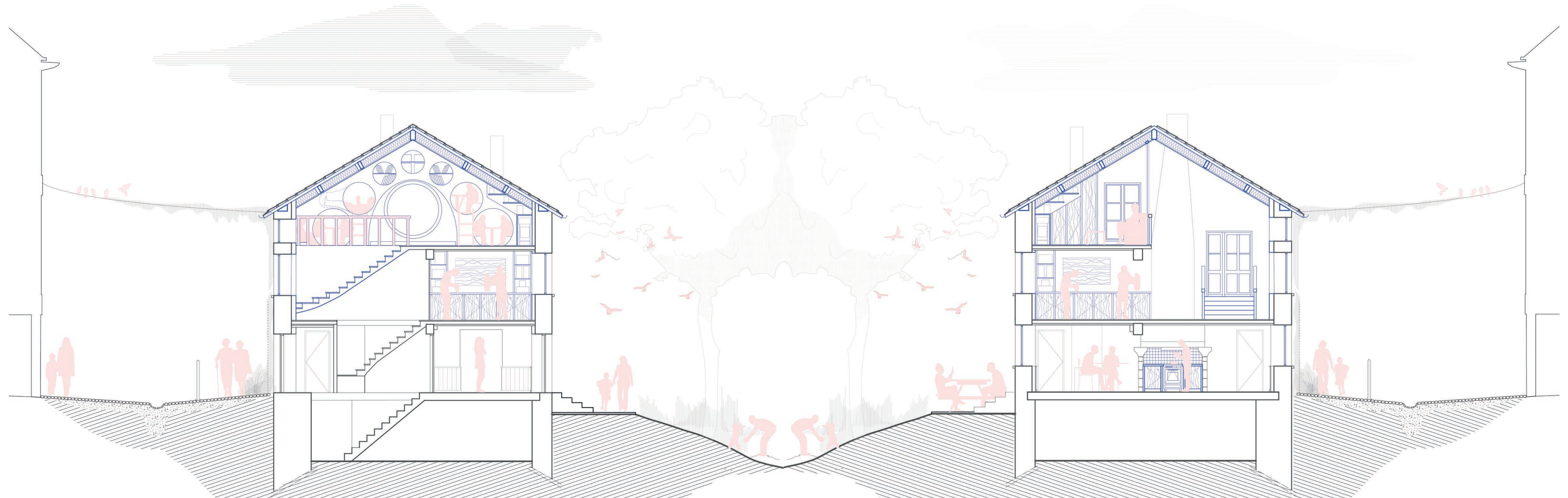
Coupe B-B' Echelle : 1/50
