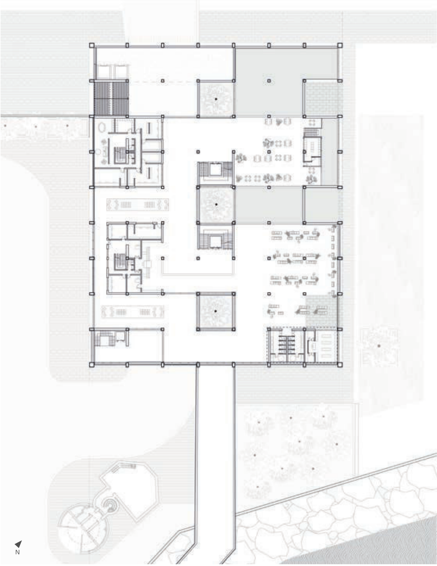
Plan de R+1, gare maritime
