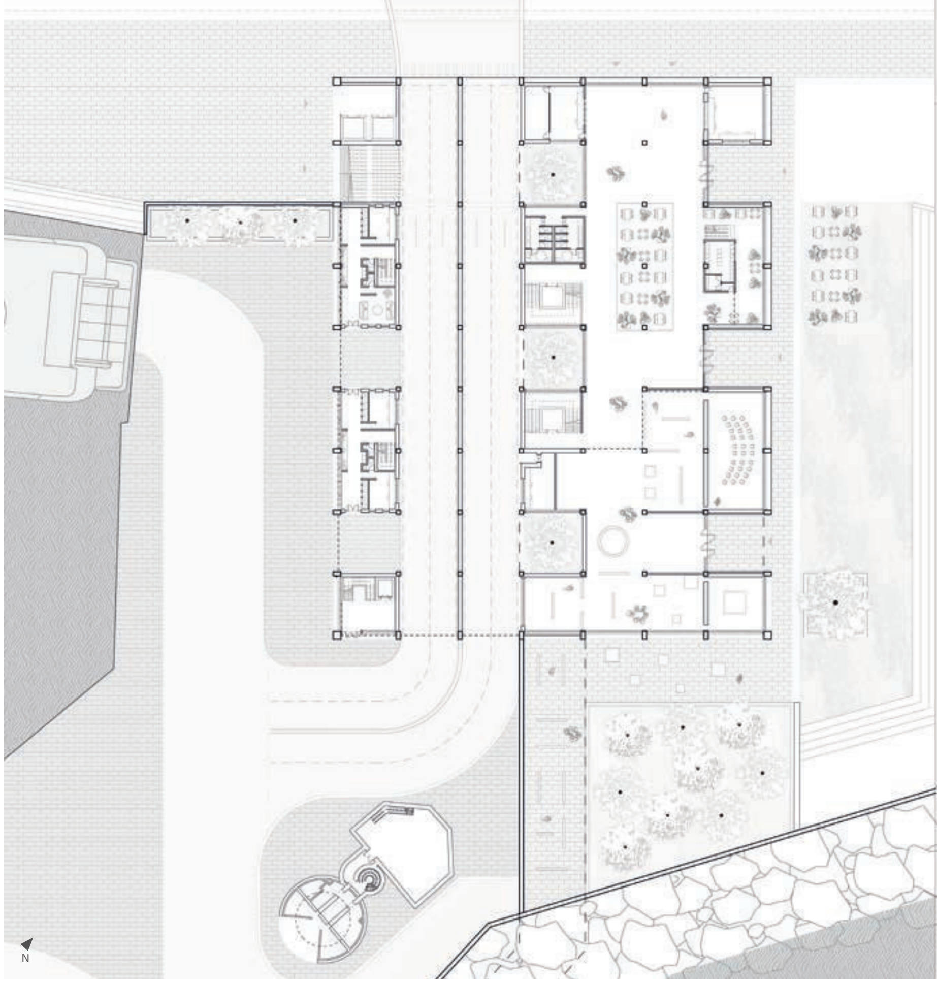
Plan de RDC, gare maritime
