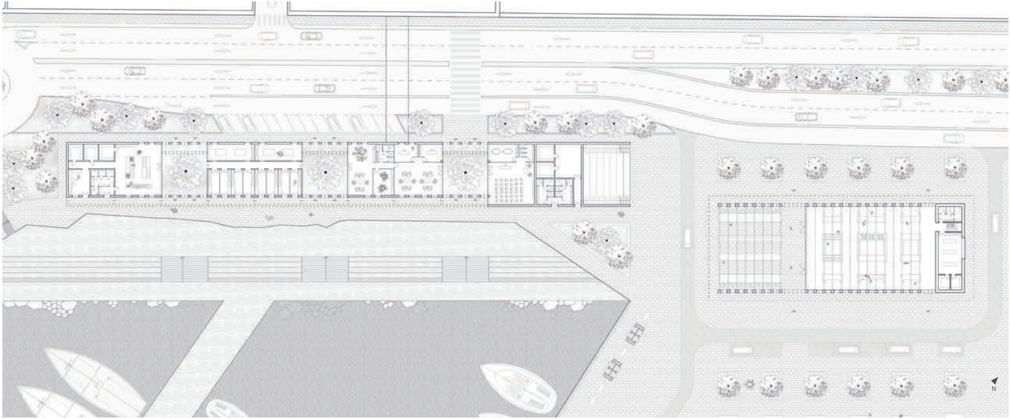
Plan de RDC, la maison des pêcheurs et la halle de marché
