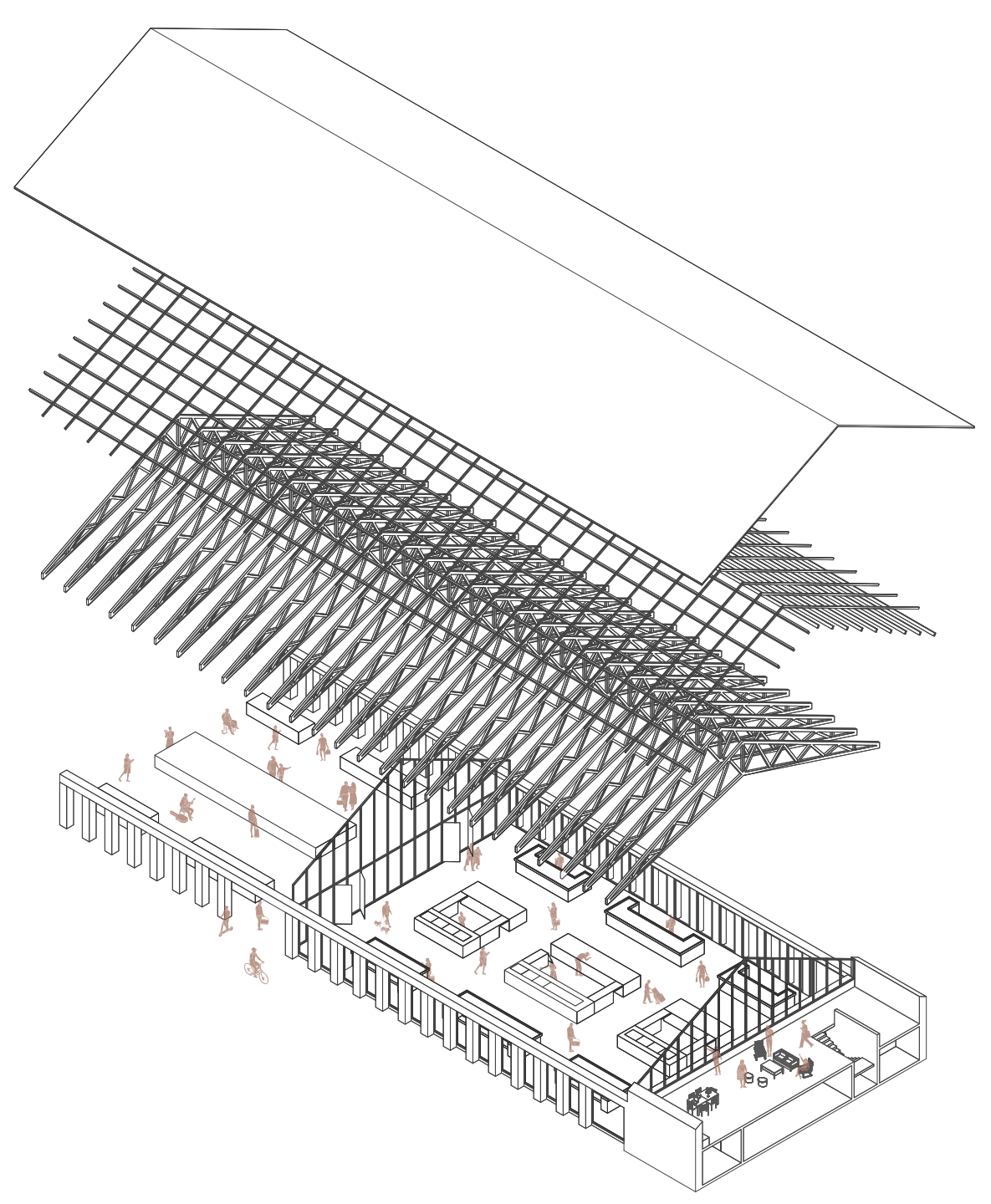
Axonométrie éclatée, halle de marché
