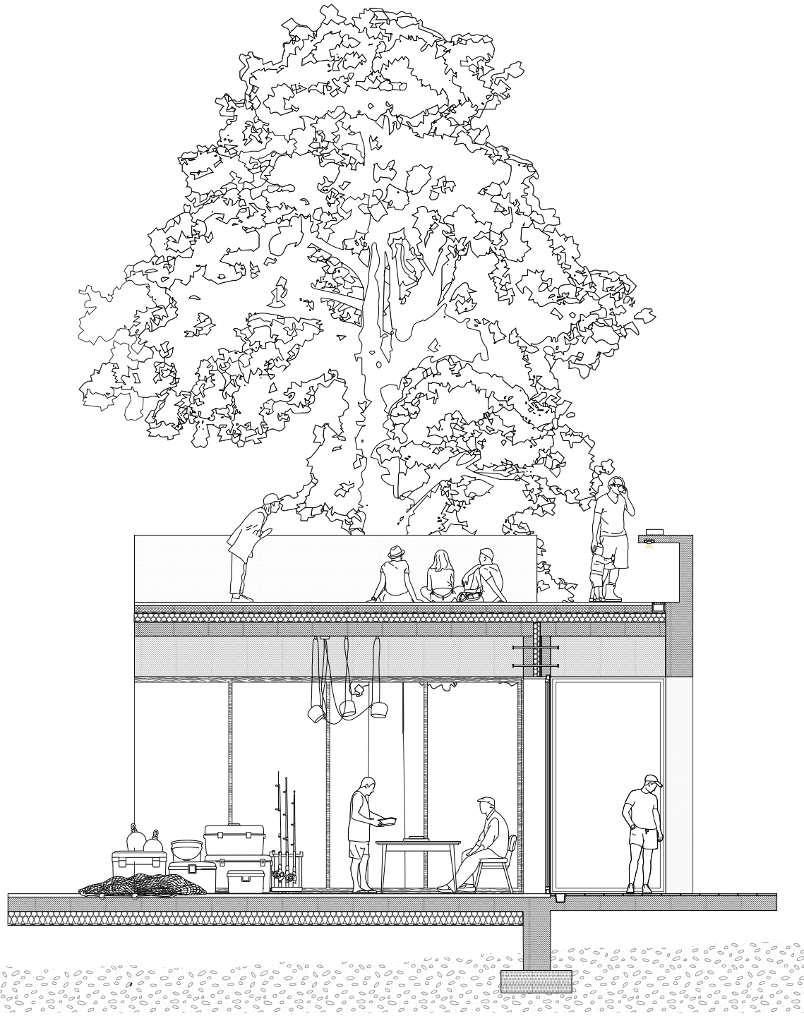
Coupe détail, maison des pêcheurs
