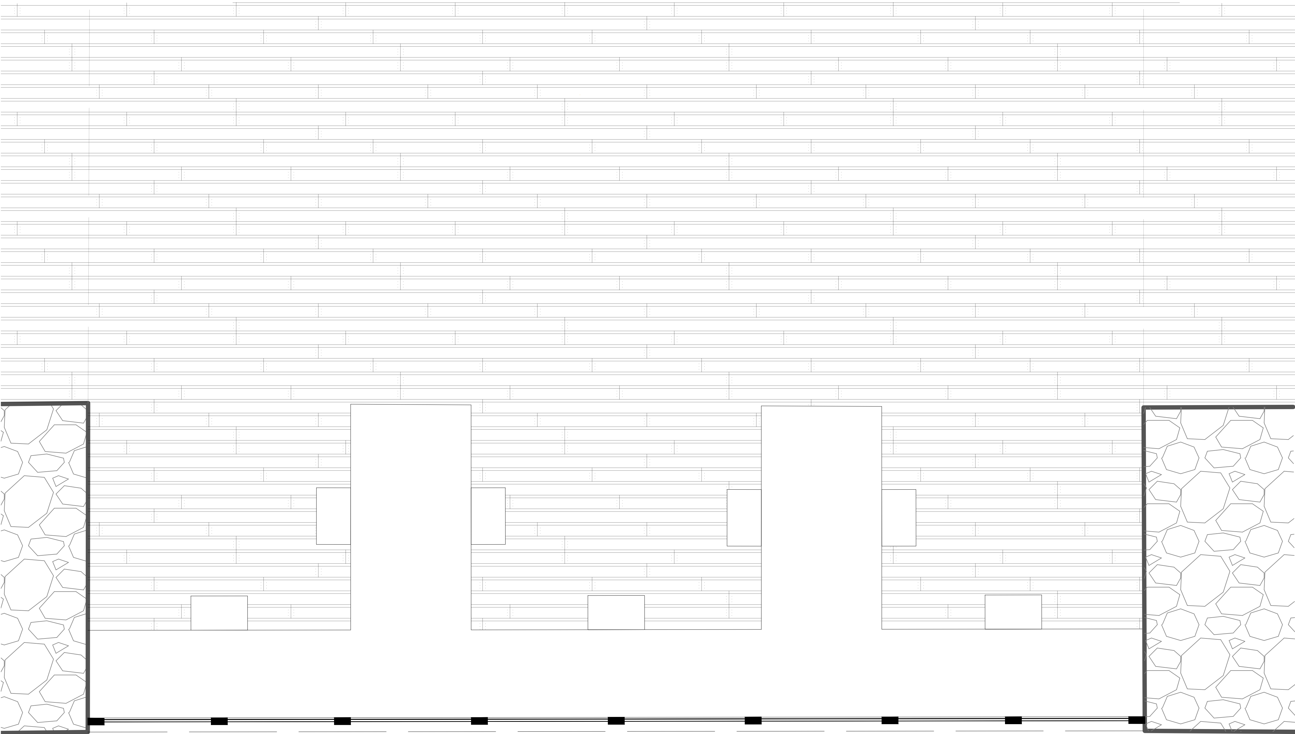
Plan de l'intérieur de la Bibliothèque des Voûtes Séquence avec cabines de réunion offrant différents niveaux d'intimité visuelle et acoustique Échelle 1:20
