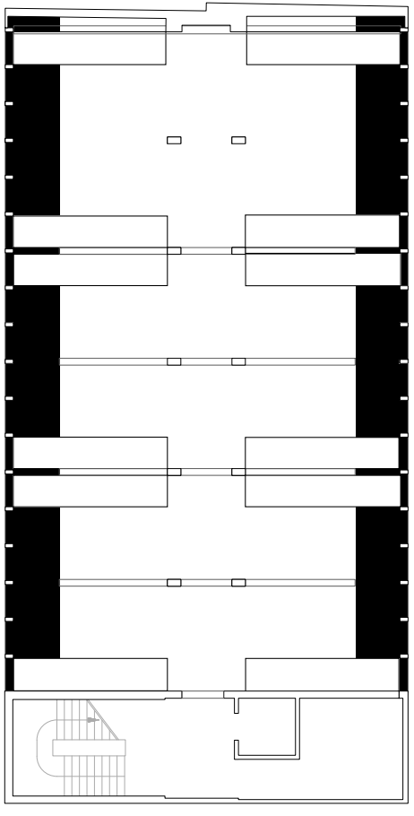
Trémis pour escalier et double hauteur
