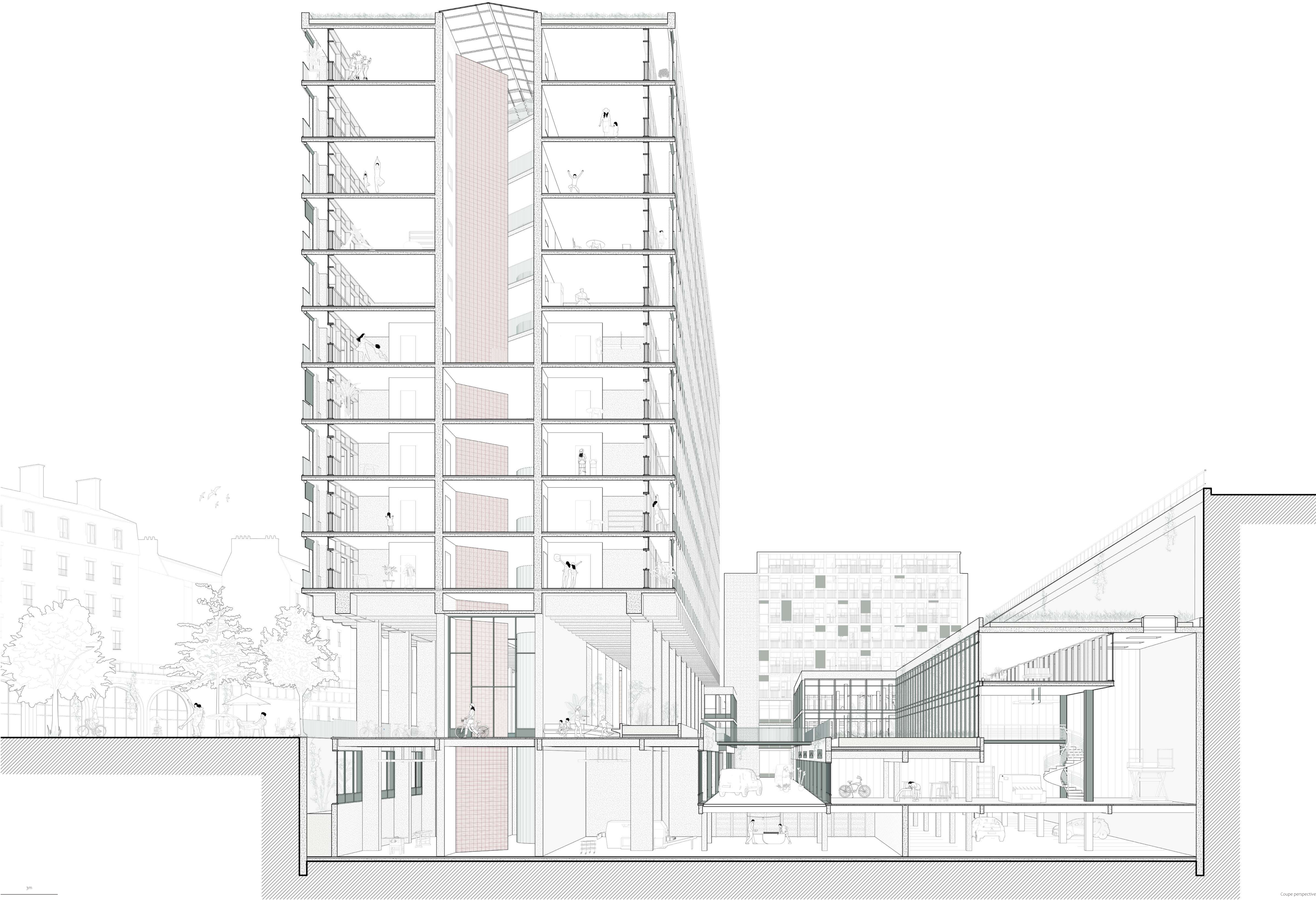
Coupe perspective
