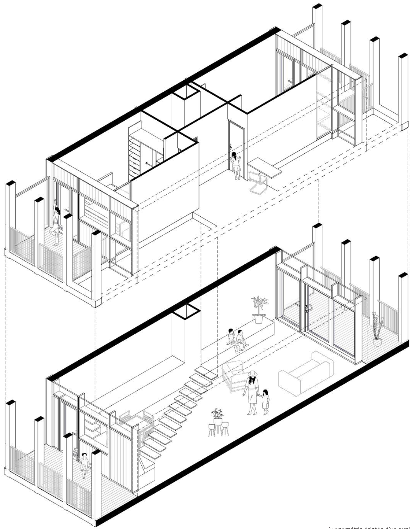
Avionnette éclairée d'un duplex
