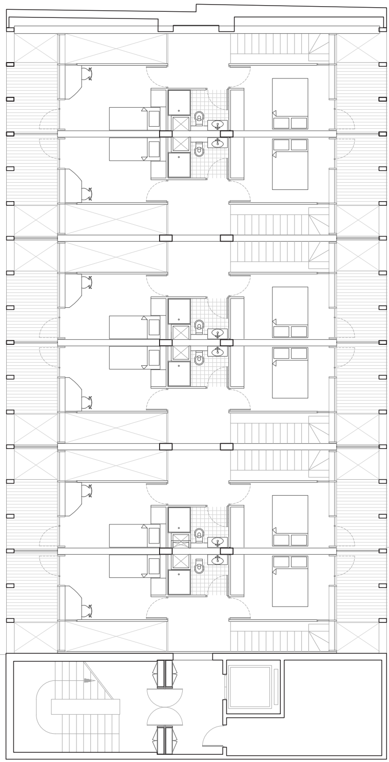
Plan bas et haut d'un duplex
