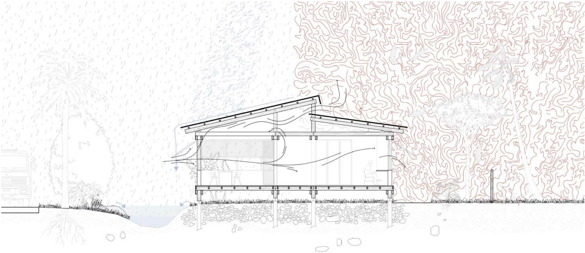
Coupe de principe - Une réponse architecturale face aux risques naturels
