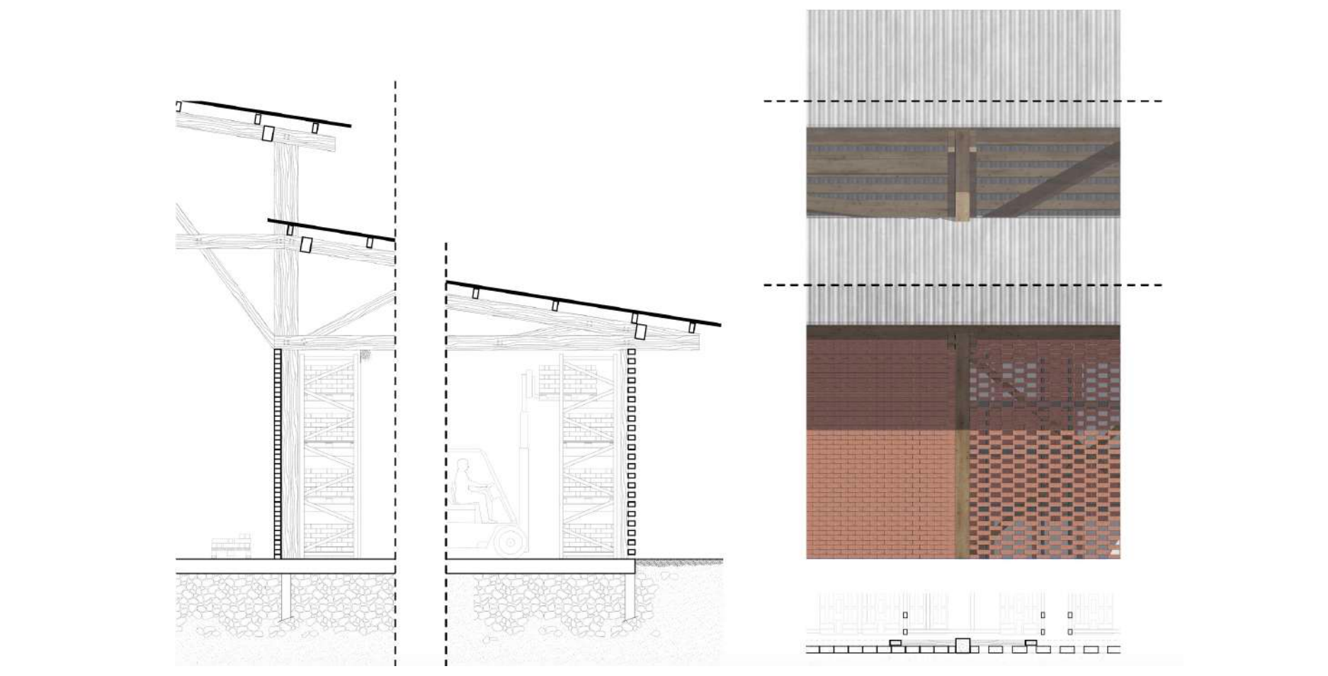
Coupe détail - Principe constructif, structure bois, remplissage brique de sargasse
