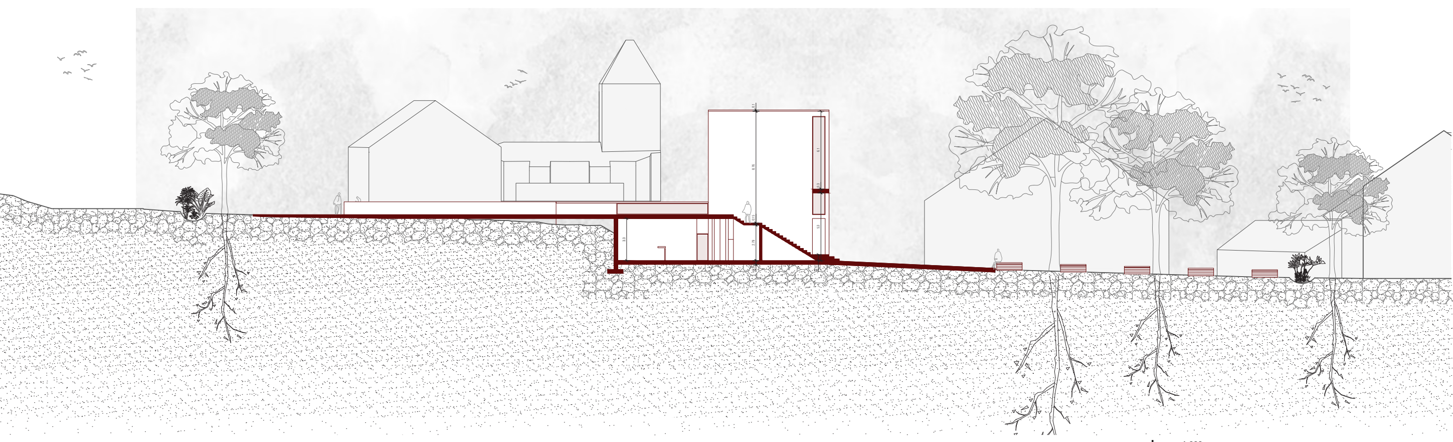
7. COUPE AA SUR LA MAIRIE
