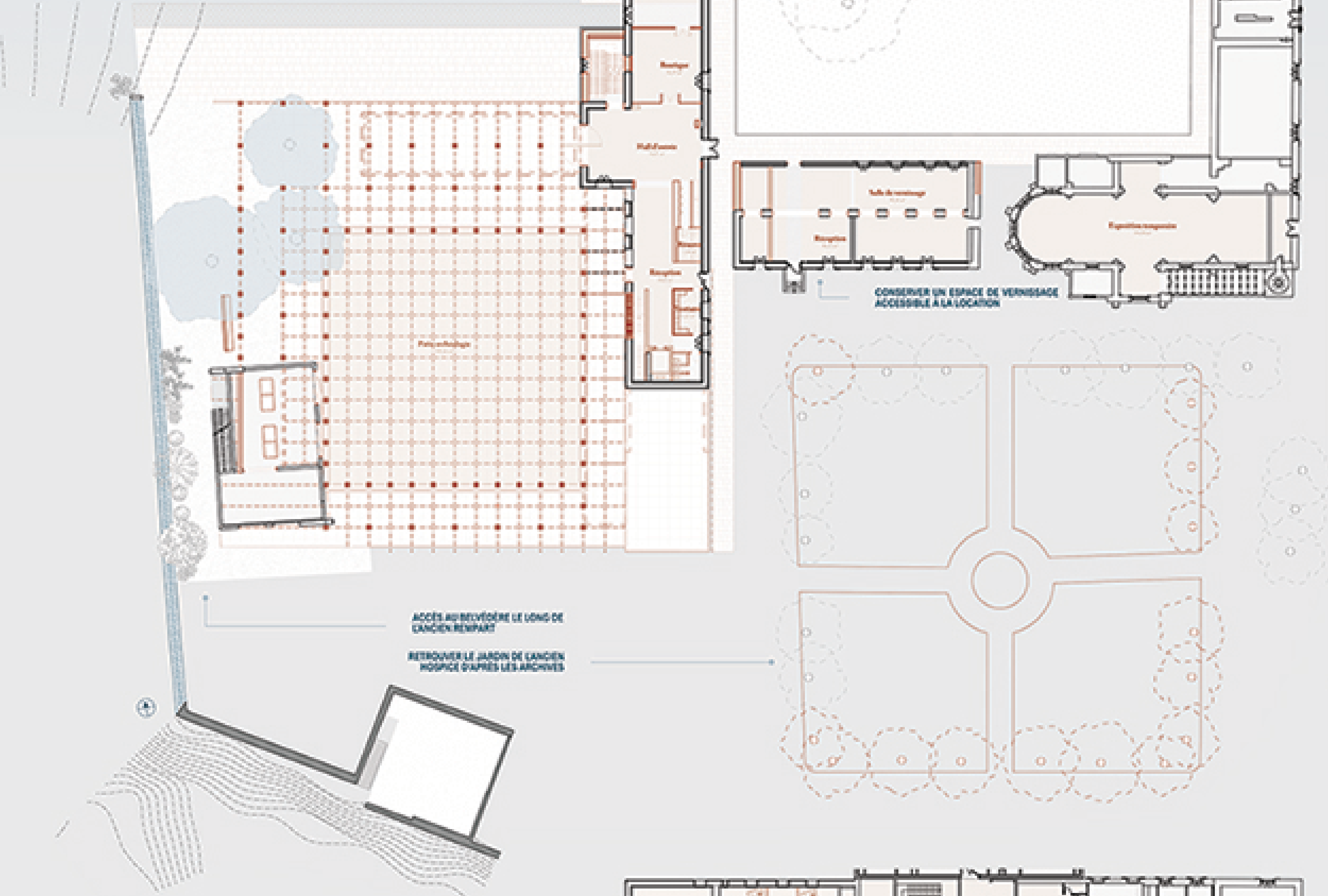
PLAN RDC DE L'ESPACE MUSÉAL 1/200 ème
