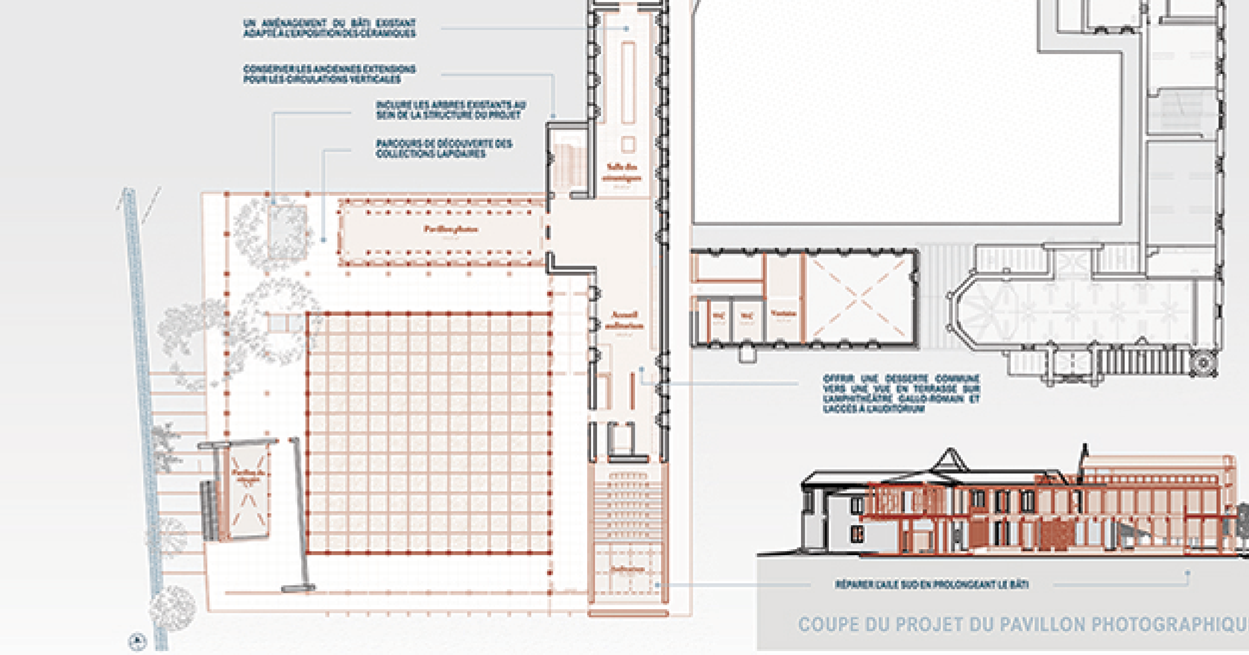
PLAN R+1 DE L'ESPACE MUSÉAL 1/200 ème
