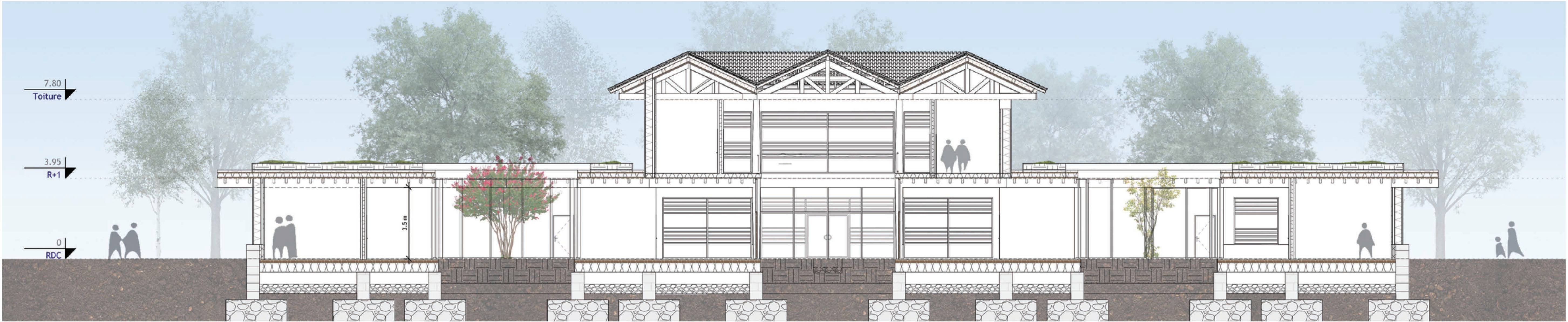
Coupe transversale AA'
