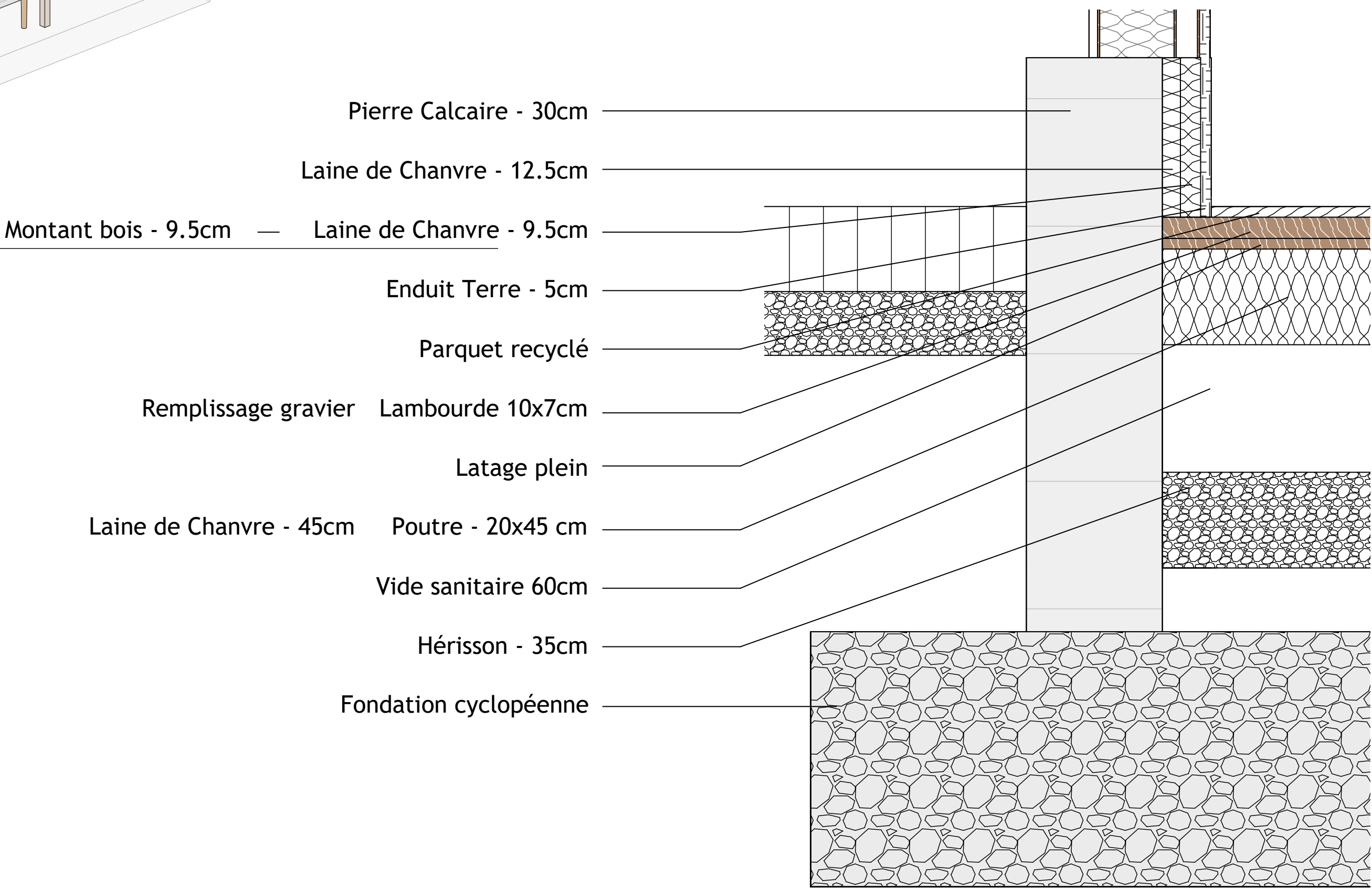
Détail dalle soubassement et mur de pierre
