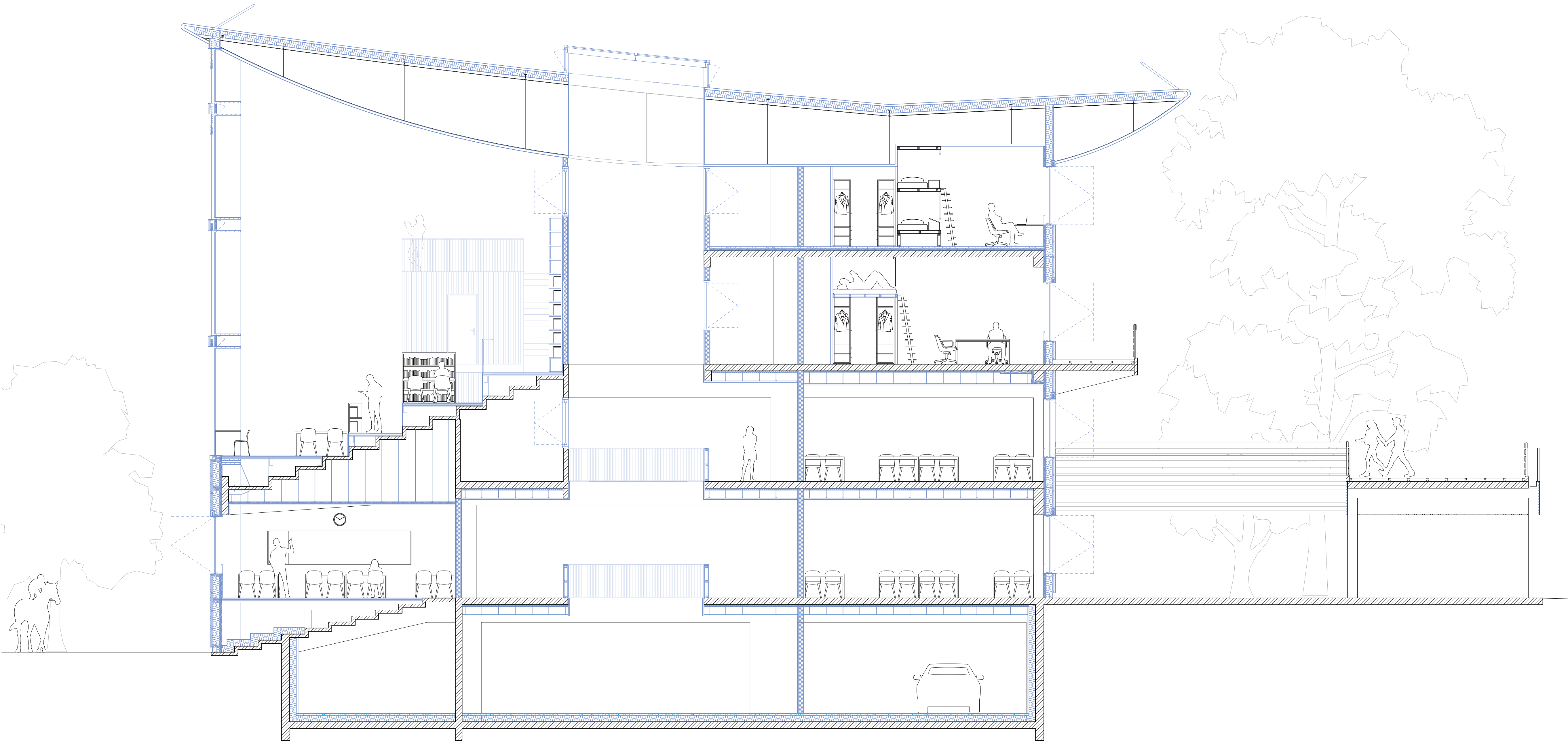
Coupe transversale - 1/50
