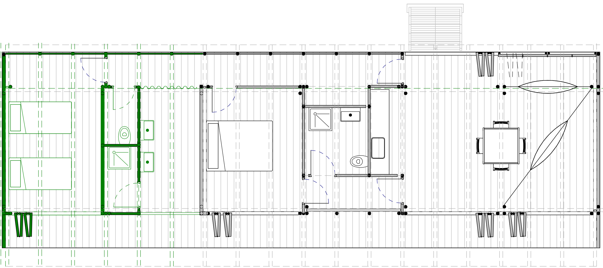
plan avant et après extension
