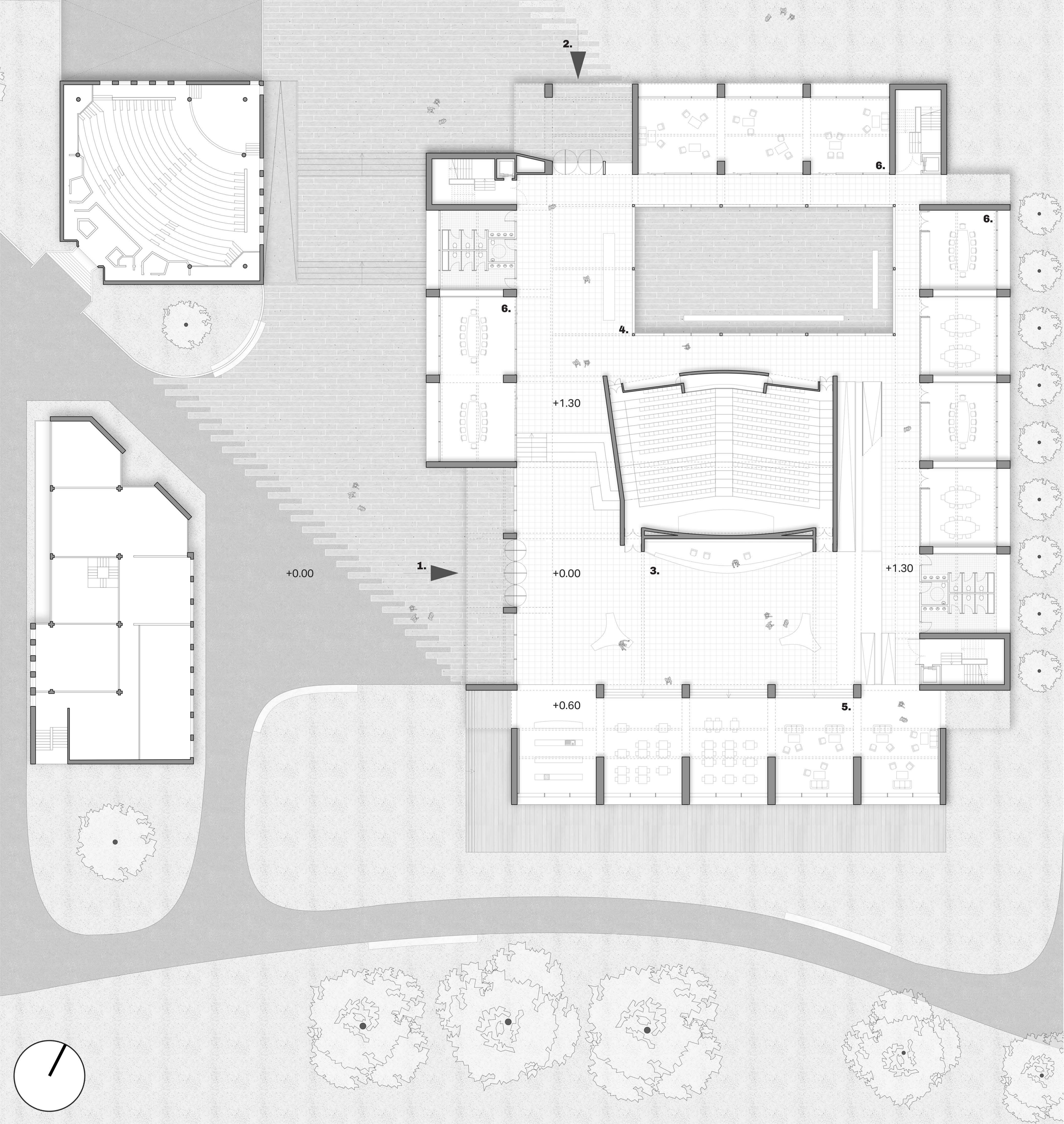
FLOOR PLAN 1 : 200
