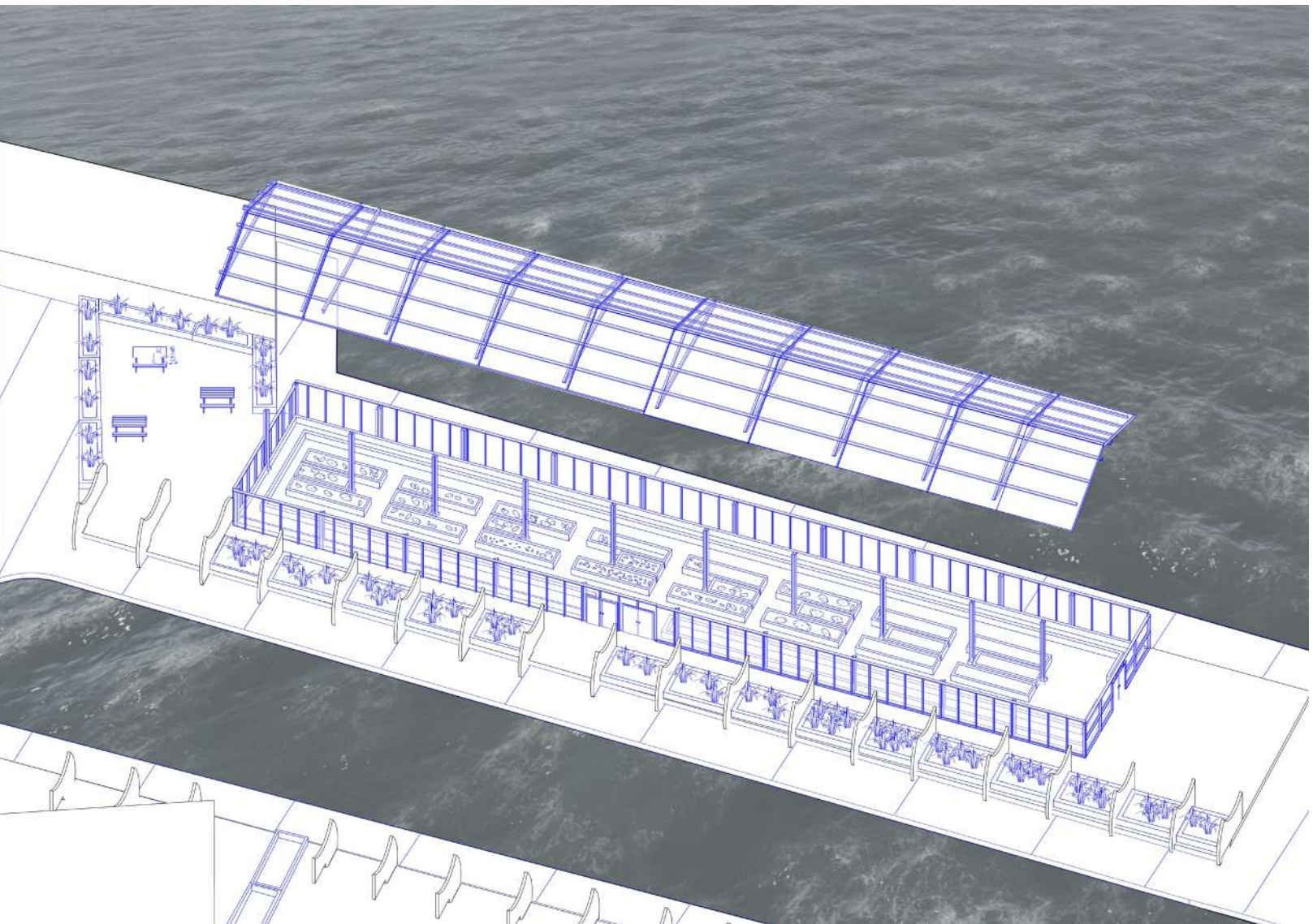
COUPE PERSPECTIVE
