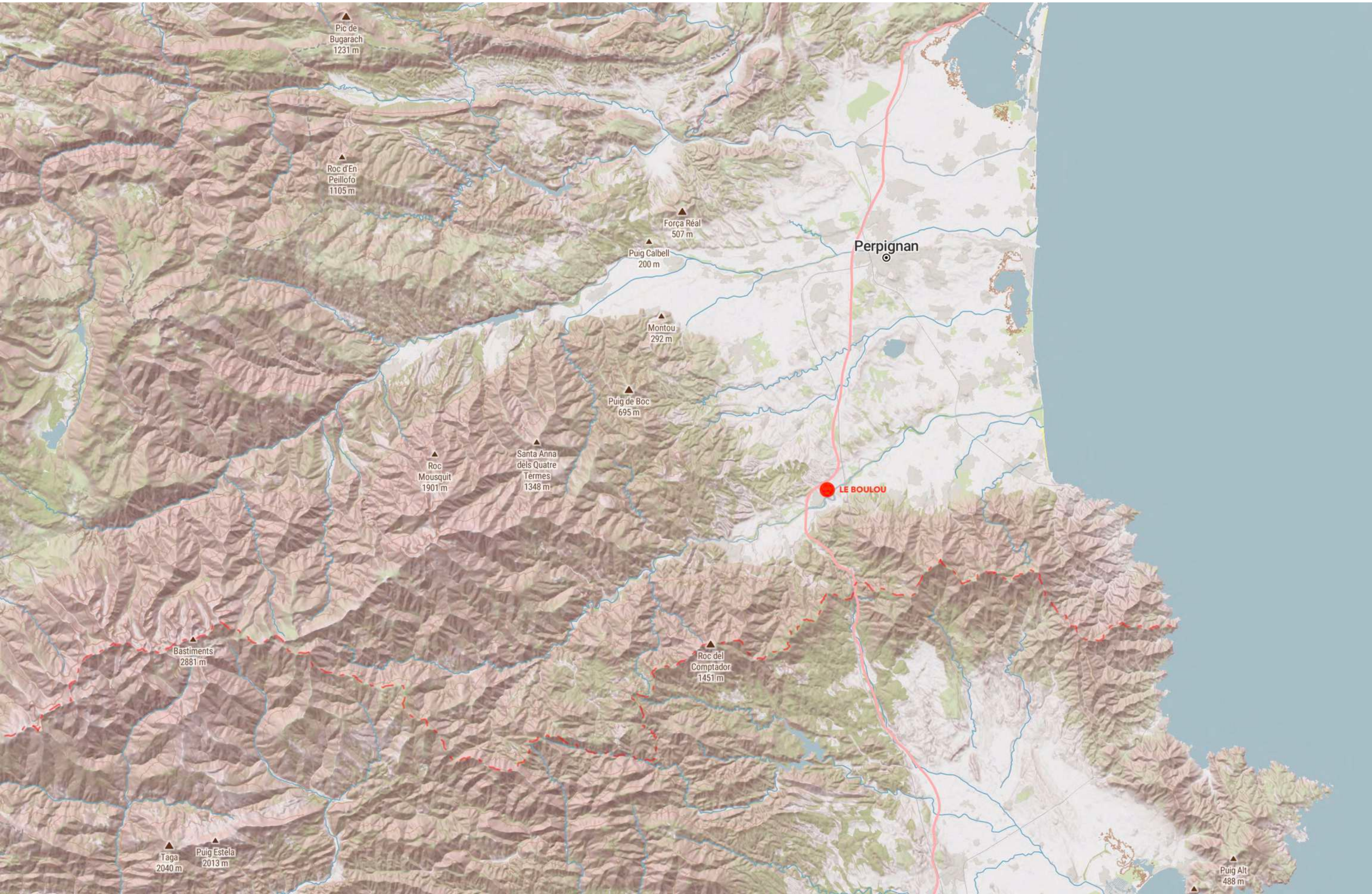
CARTE TOPOGRAPHIQUE 1:200000
