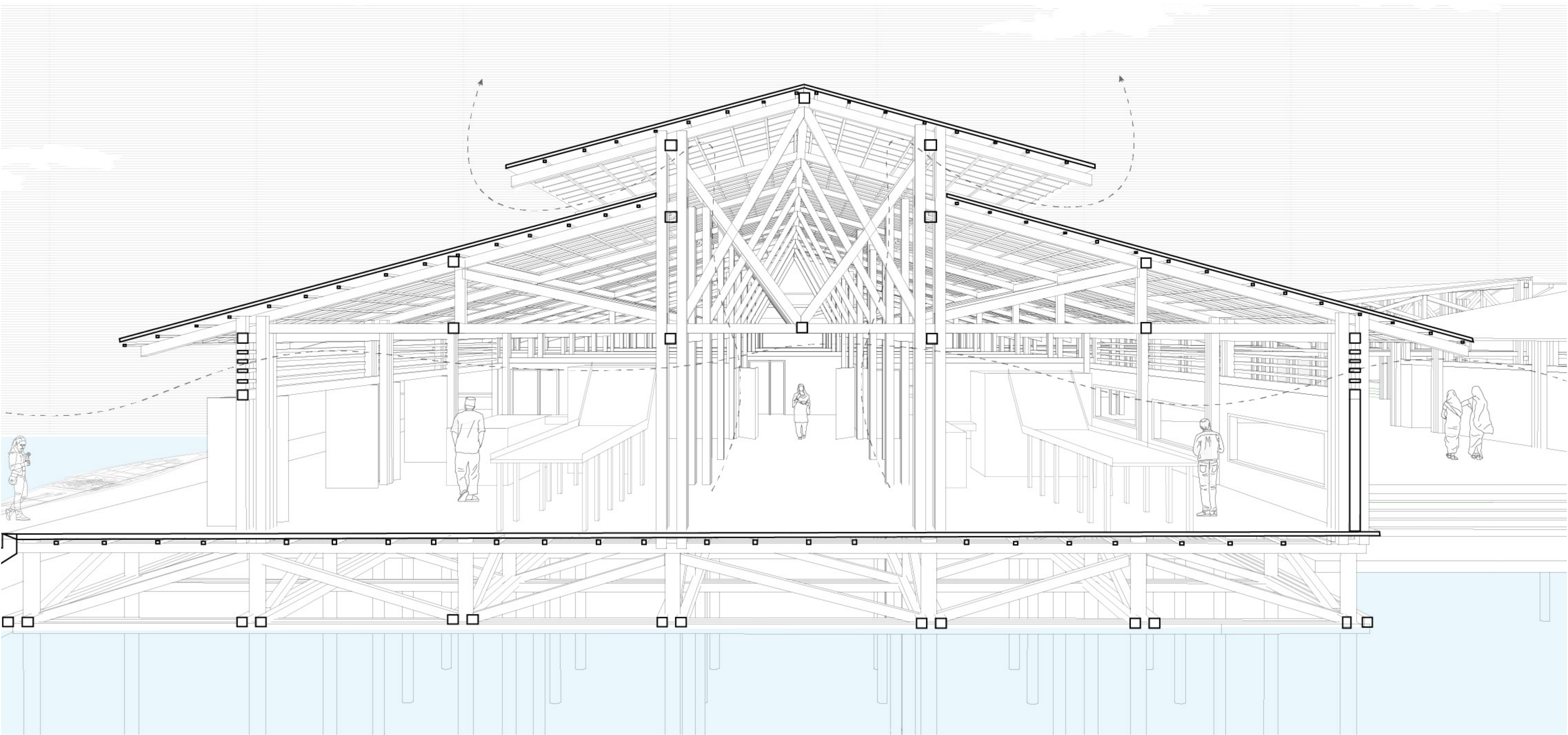
coupe perspective
