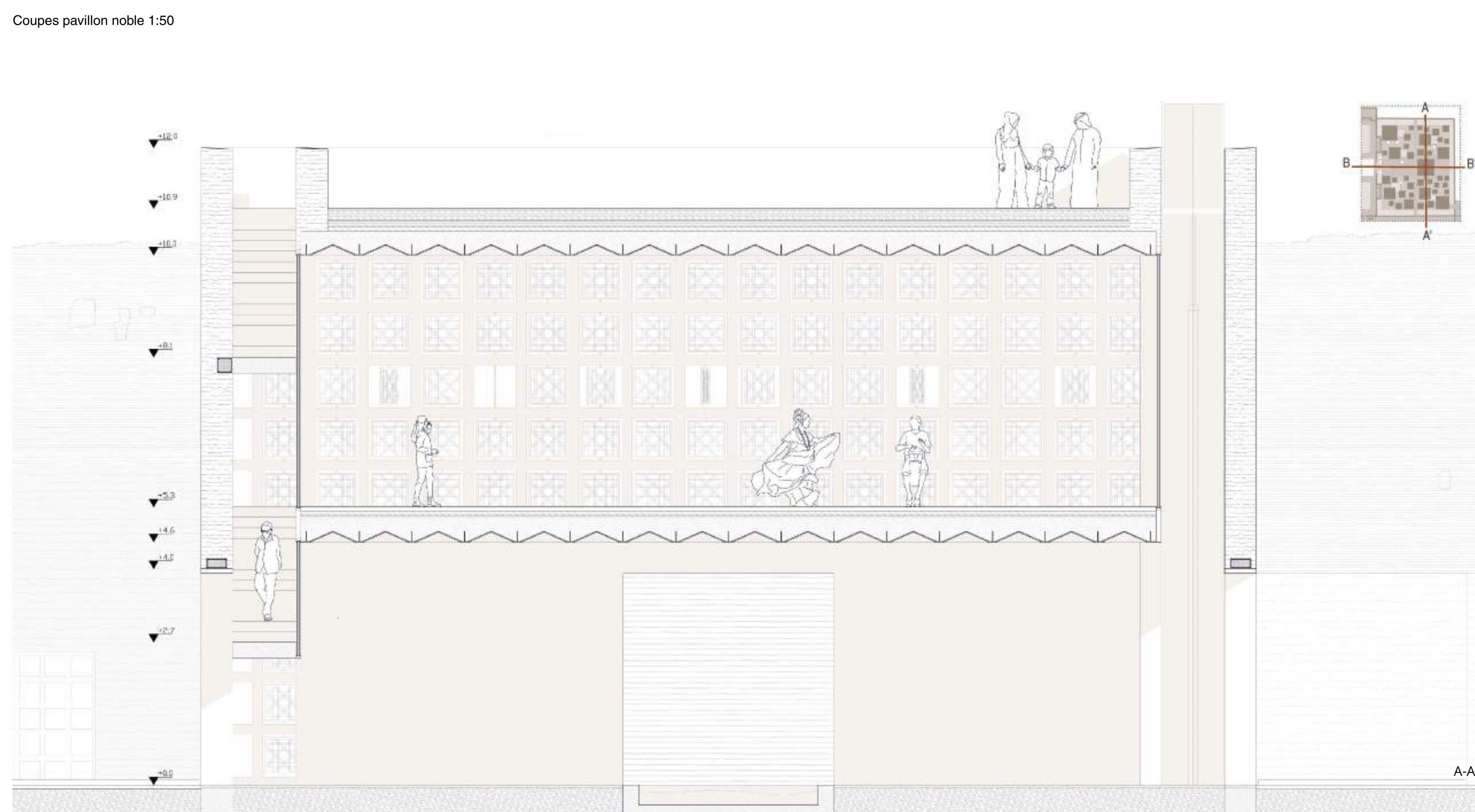
Coupes pavillon noble 1:50
