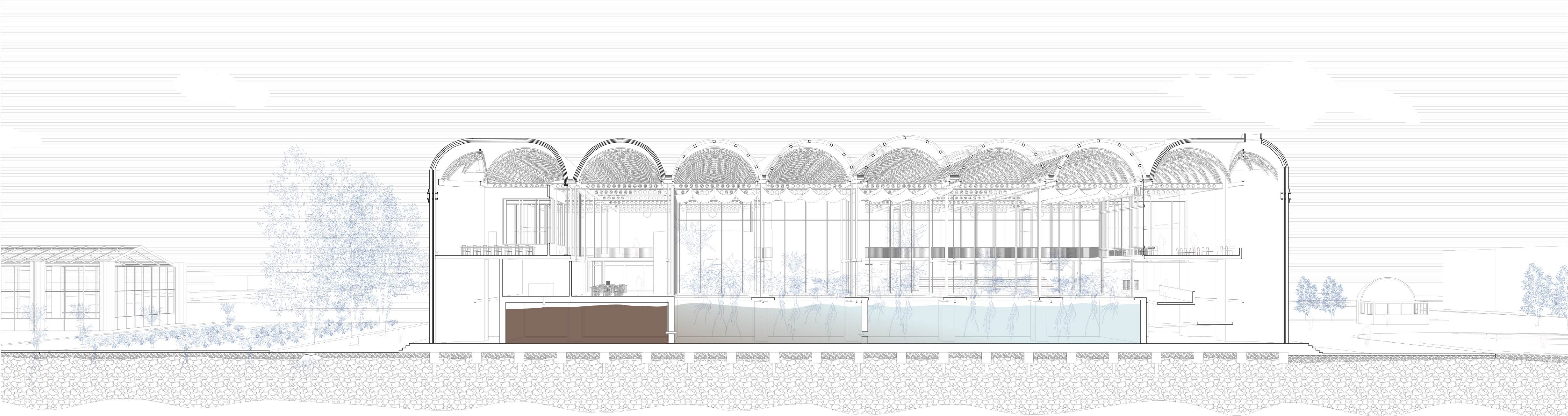
Coupe perspective 1/200ème
