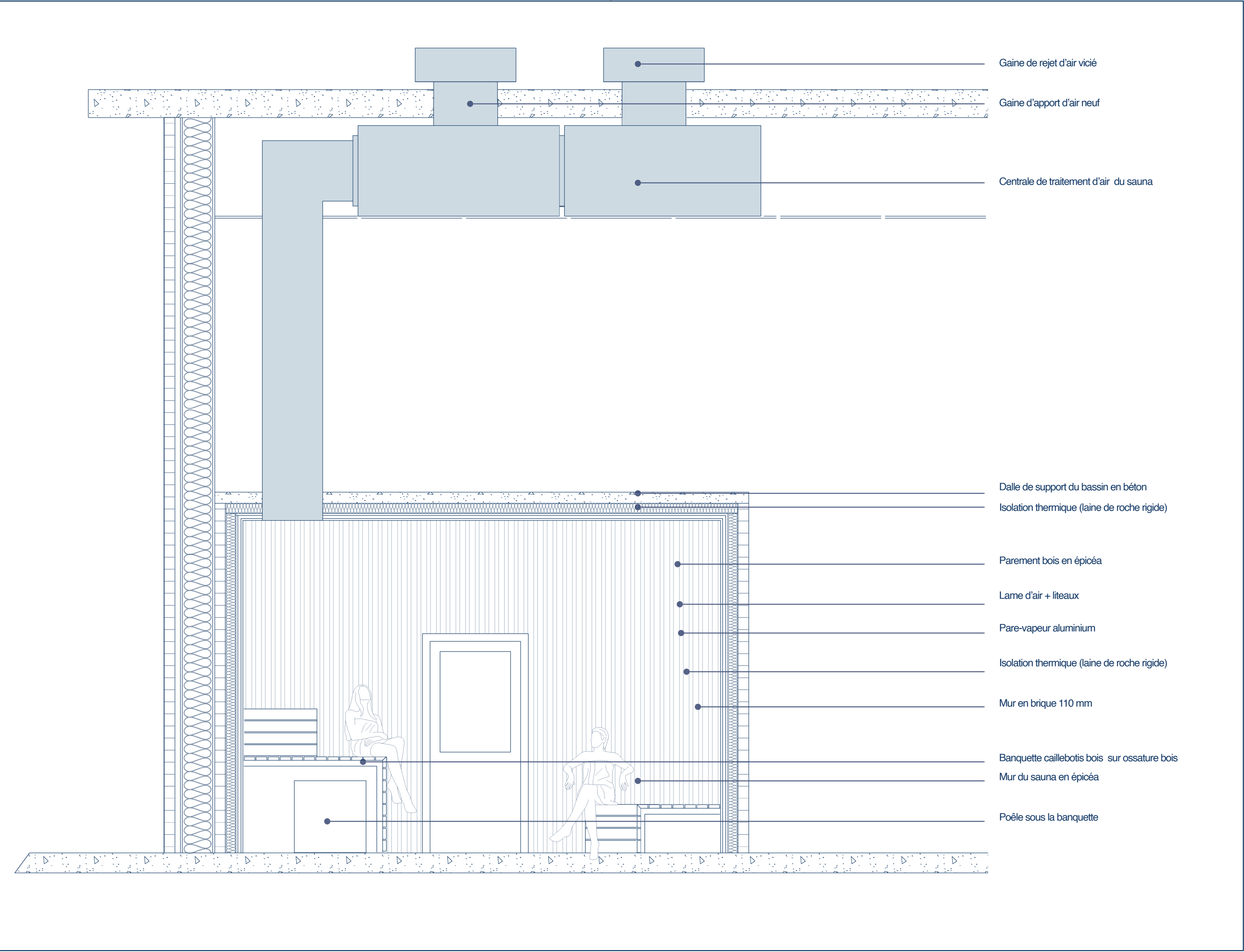
Détail Technique du sauna
