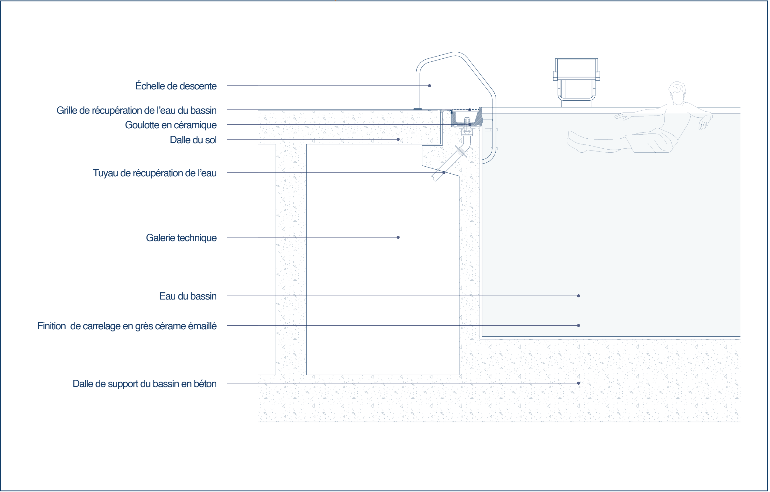
Détail Technique du bassin
