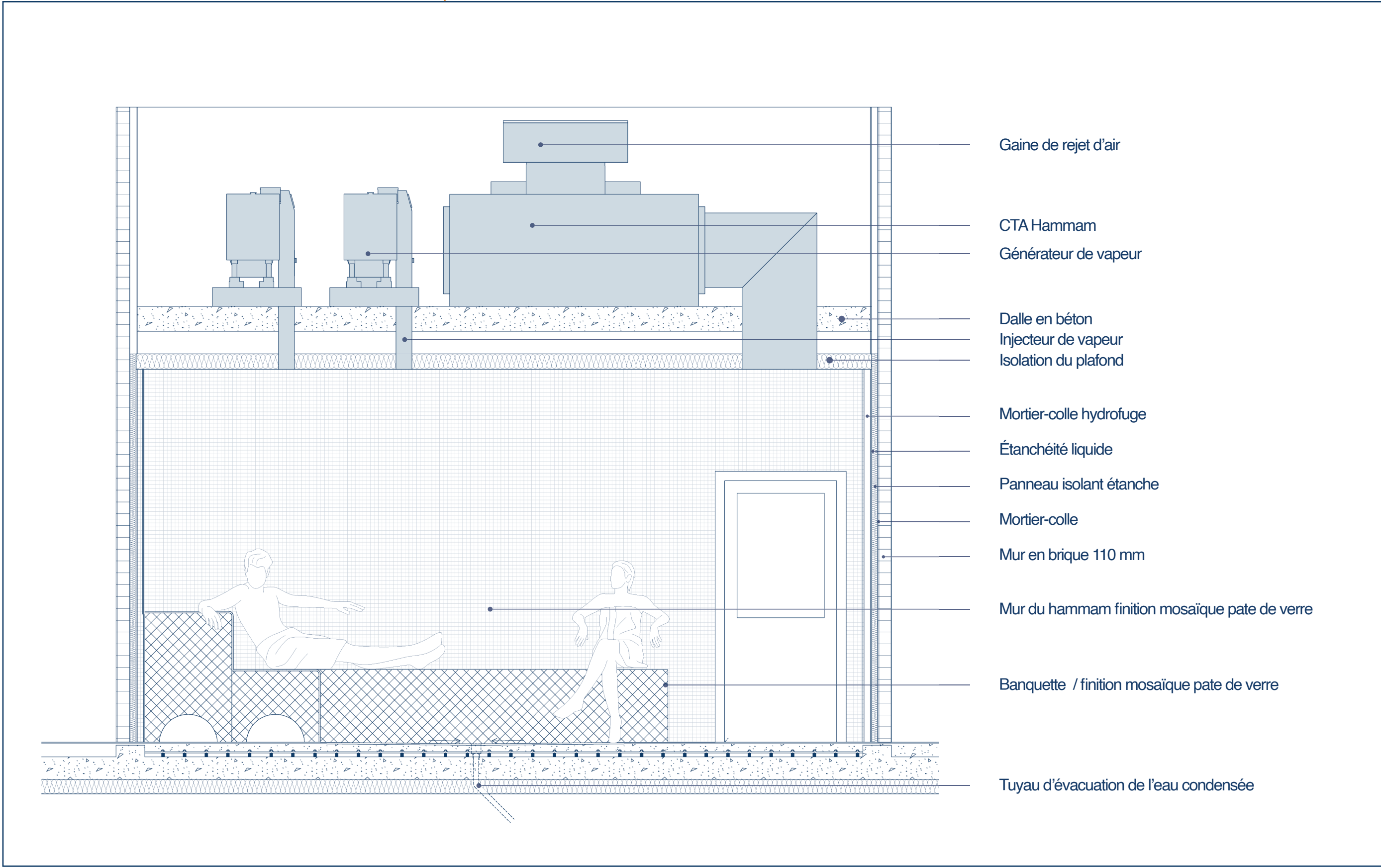
Détail Technique du Hammam
