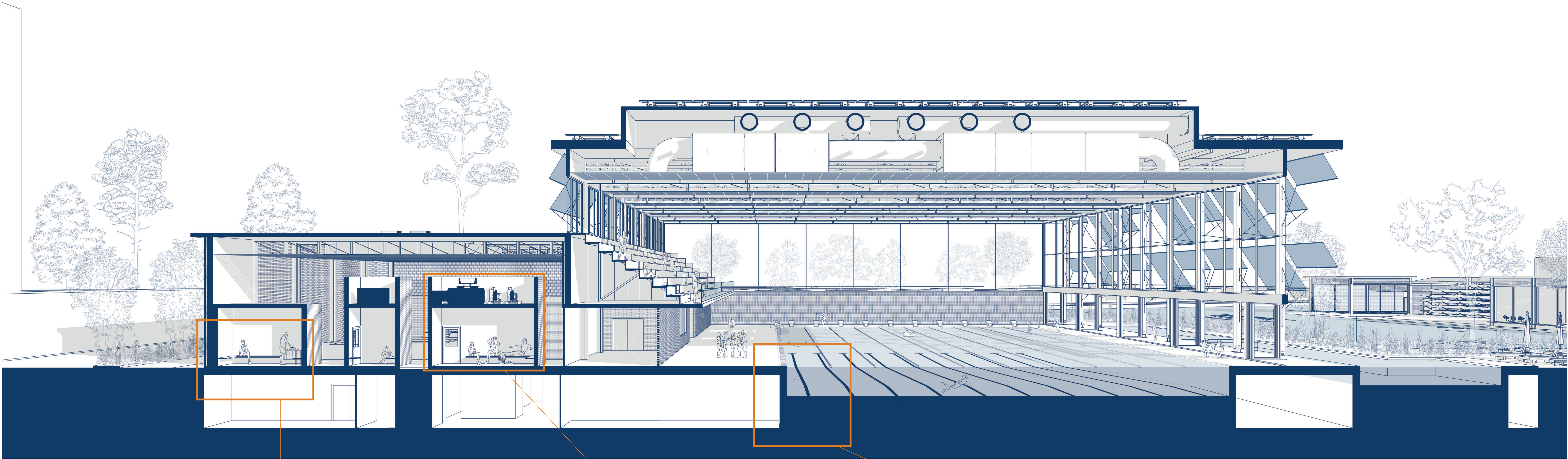
Coupe perspective Ouest - Est
