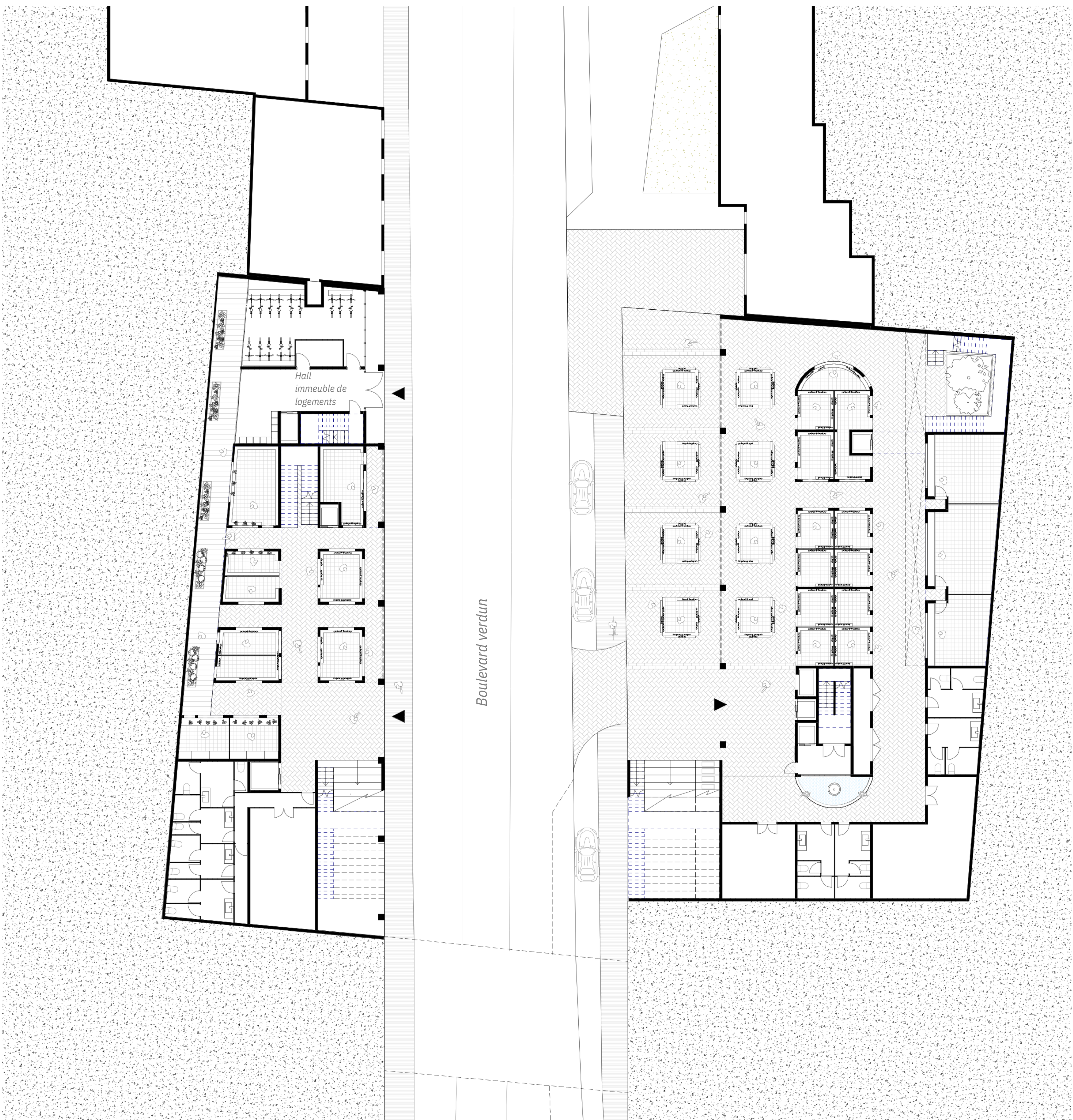
PLAN NIVEAU VERDUN 1/200
