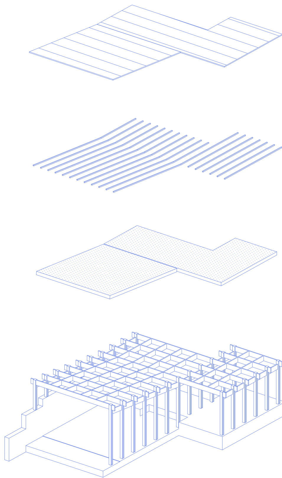
Axonométrie éclaté
