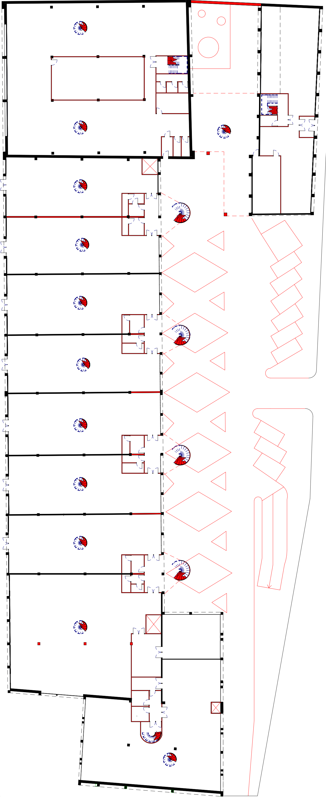
Plan déconstruction RDC
