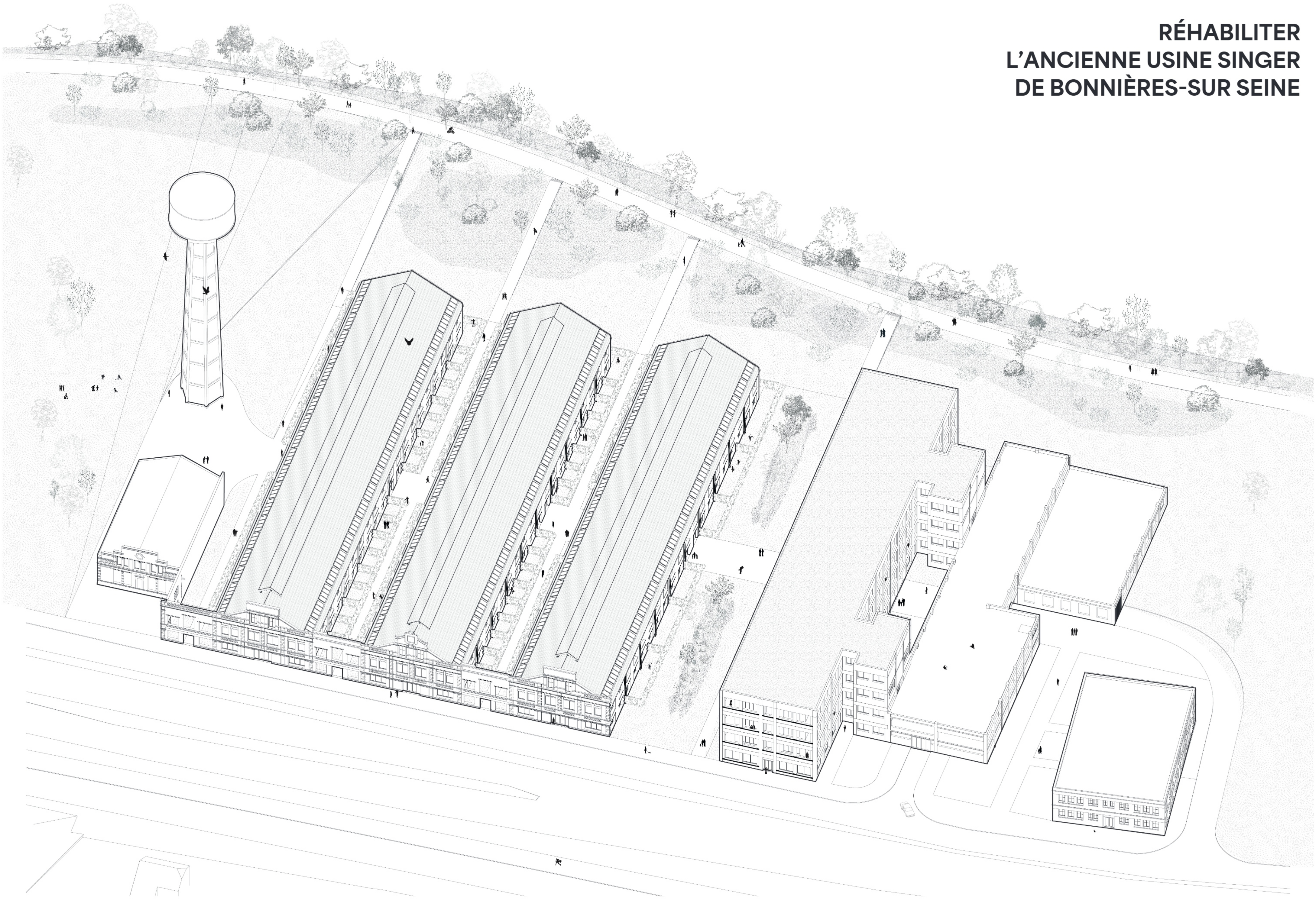
Axonométrie du projet
