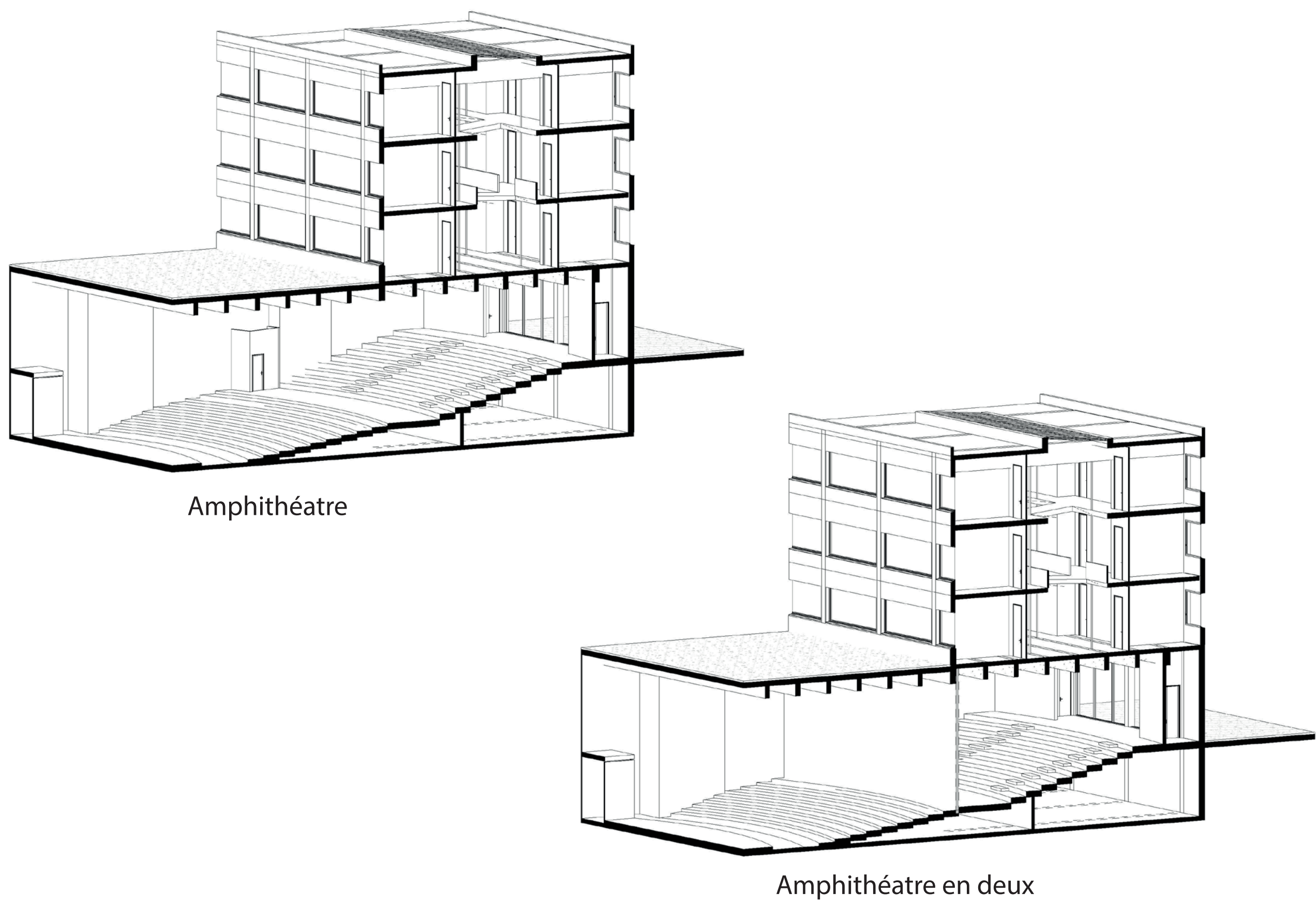
Modularité de l'amphithéâtre
