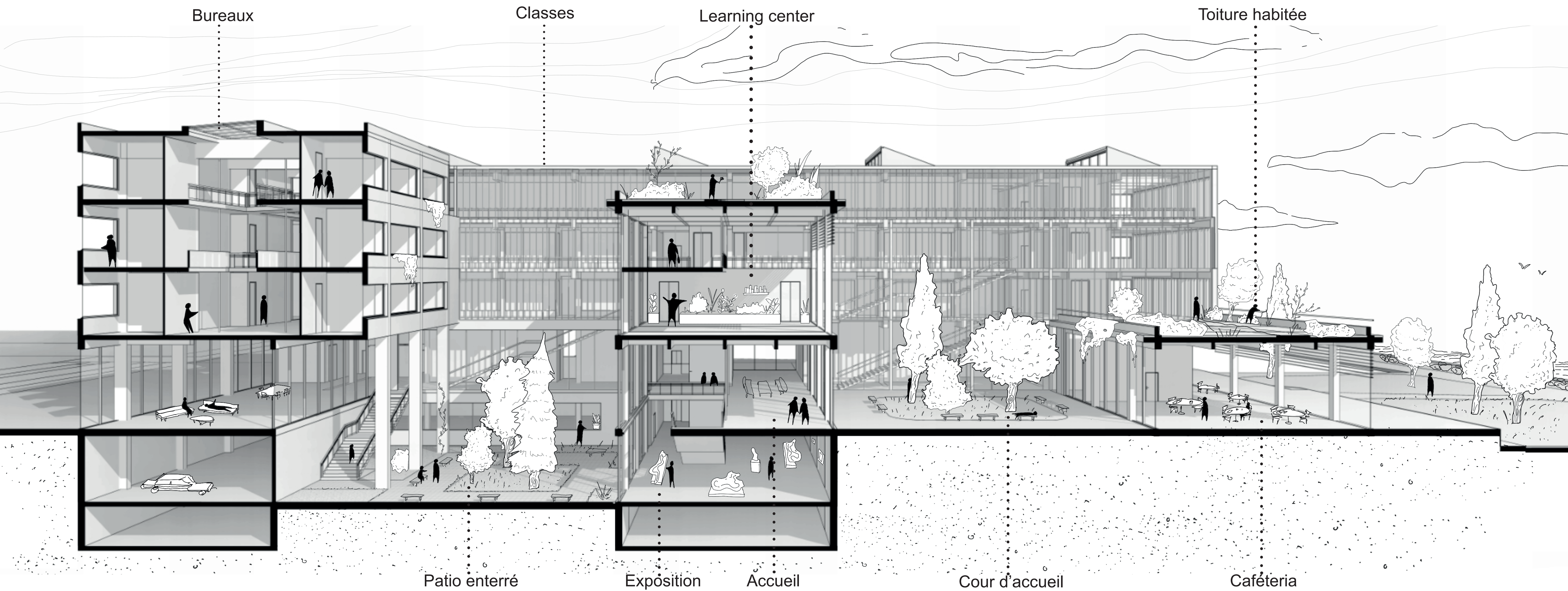
Coupe Longitudinale
