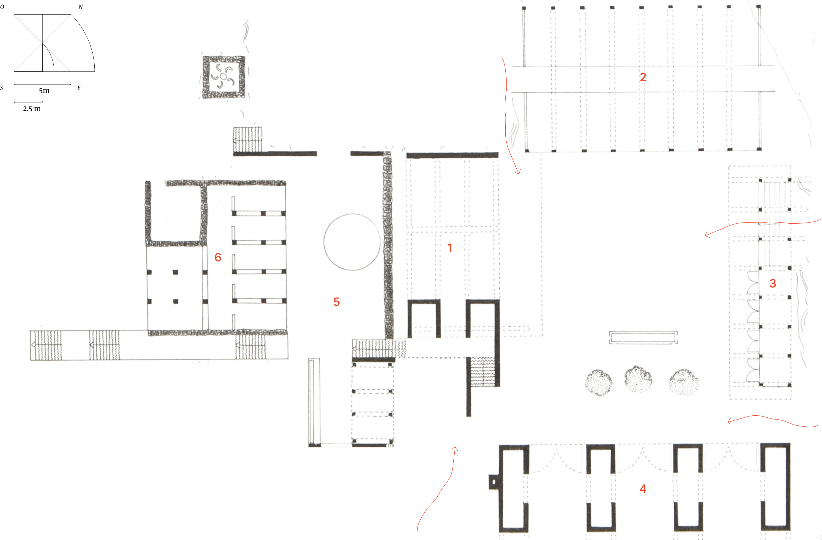
Fig 05 ci-contre : Plan du projet 1 : 200 Fig 06 ci-dessous : coupe longitudinale 1:150
