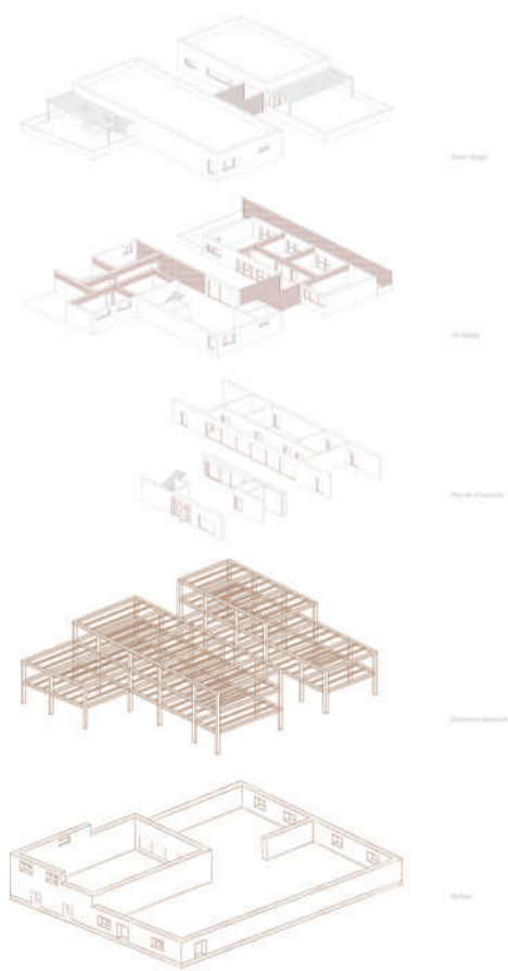
Axonométrie éclatée du centre médical et sa structure
