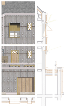
Façade en cœur d'îlot
