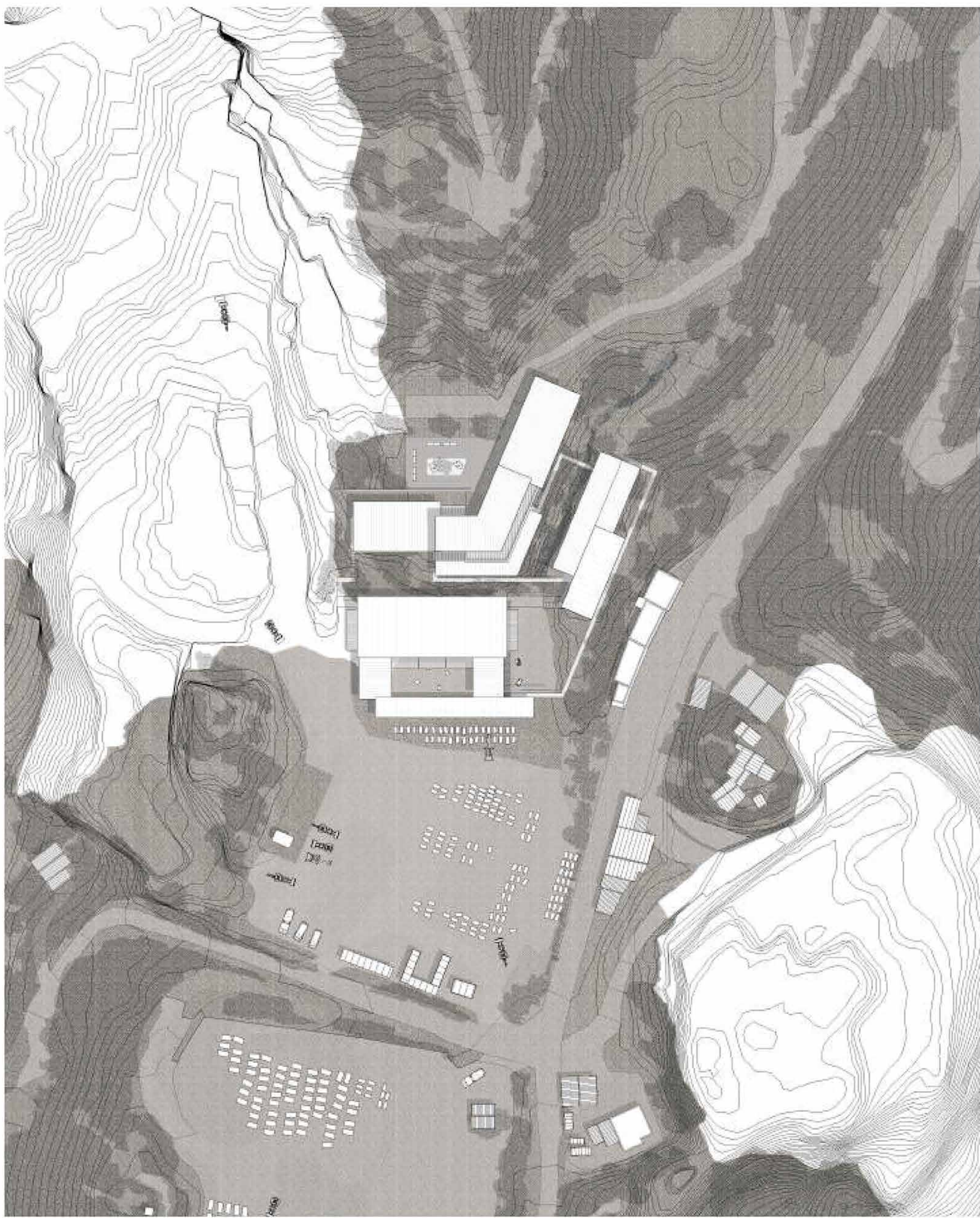
PLAN MASSE - 1/750ème
