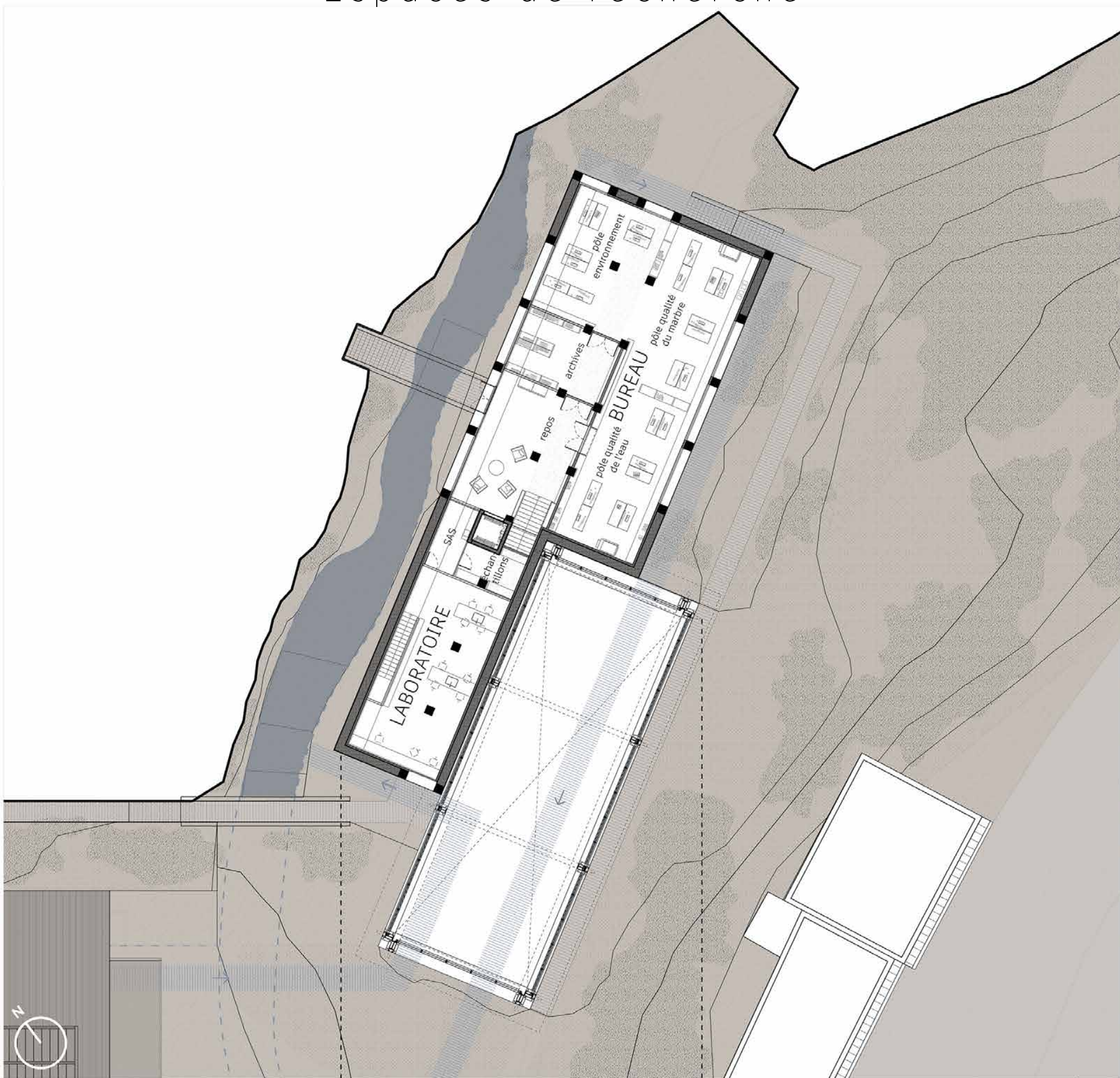
PLAN LABORATOIRE - 1/250ème
