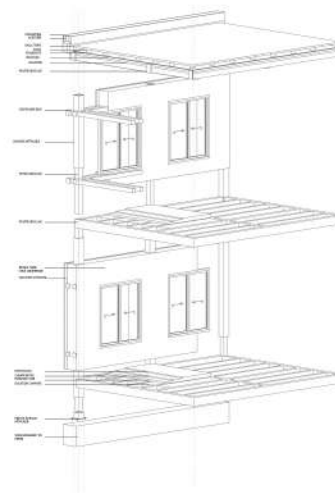
PRINCIPE CONSTRUCTIF
