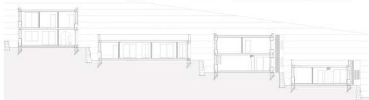
COUPE PAYSAGÈRE - GÉSTION & STABILISATION DE LA PENTE
