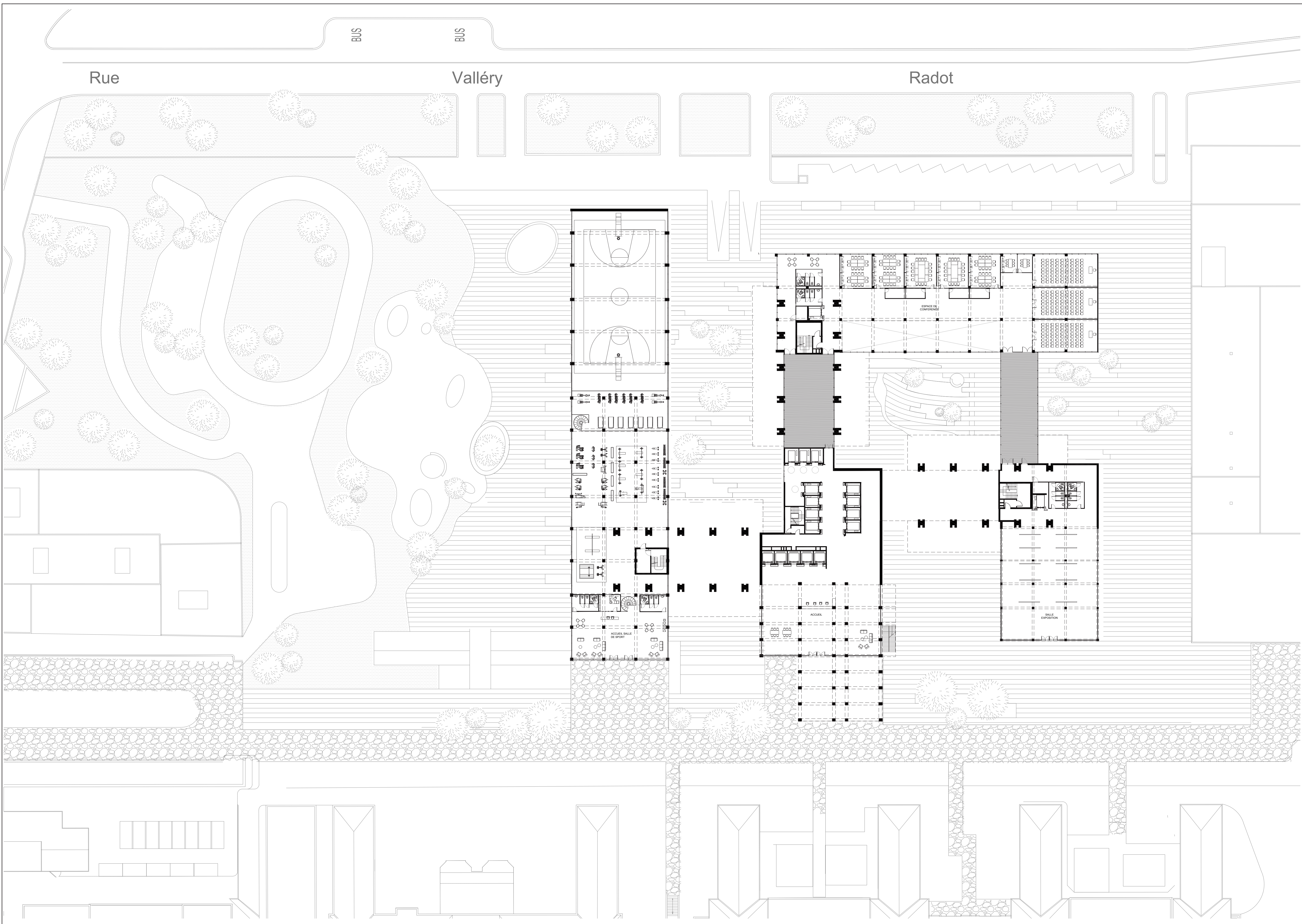
PLAN RDC ÉCHELLE : 1/333
