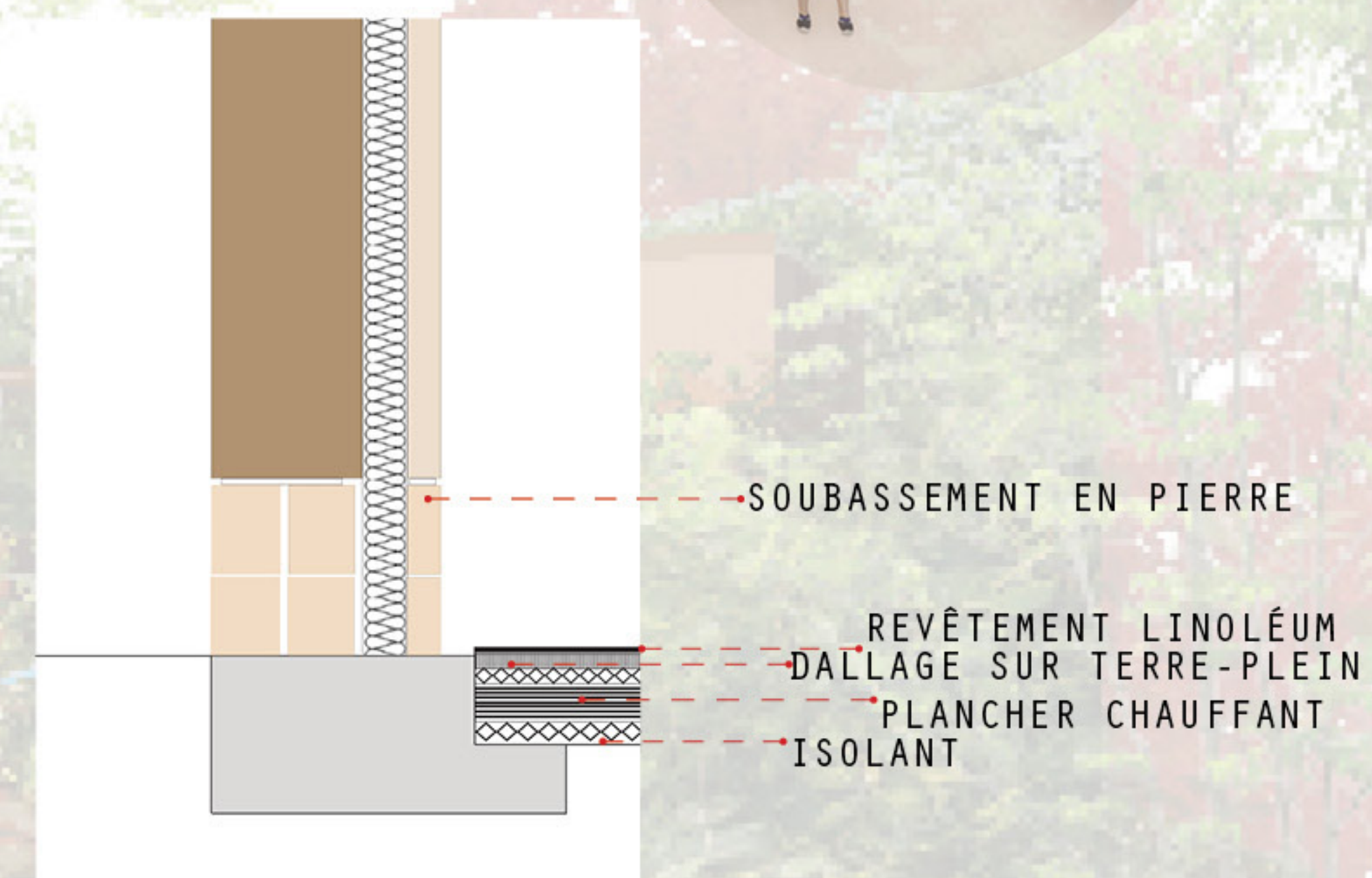
DÉTAIL COUPE PLANCHER
