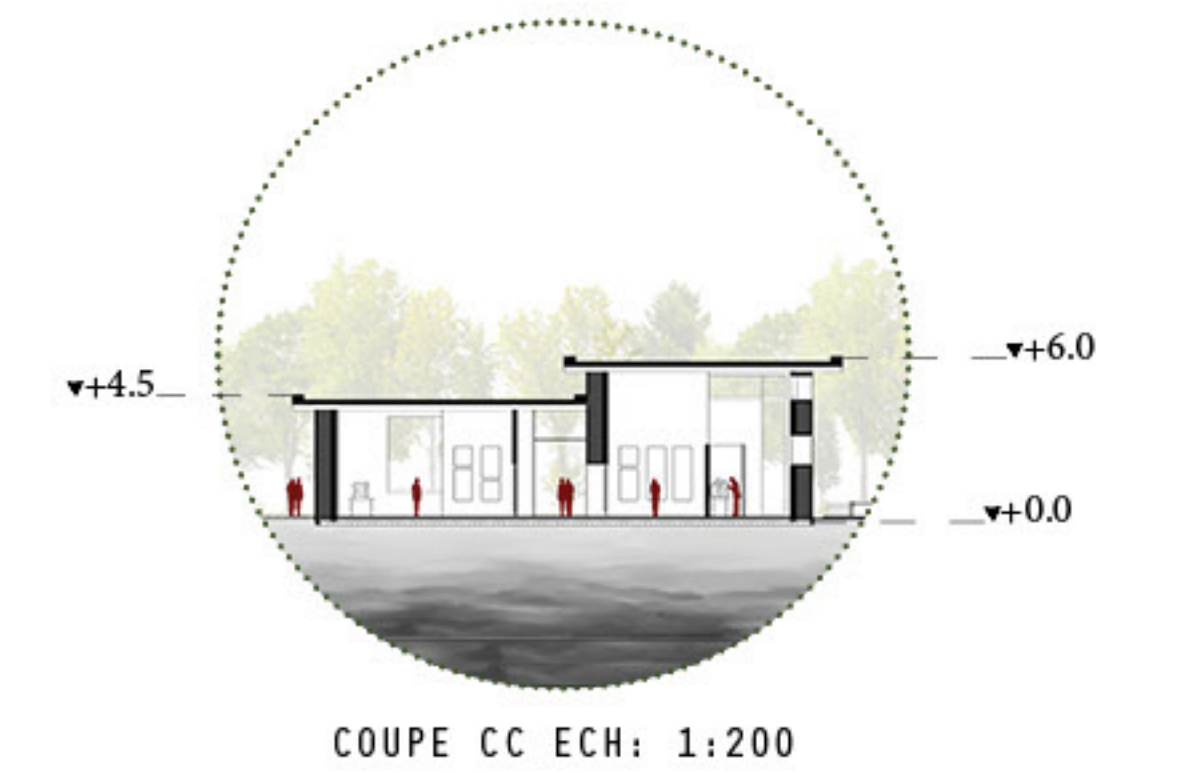
COUPE CC ECH: 1:200
