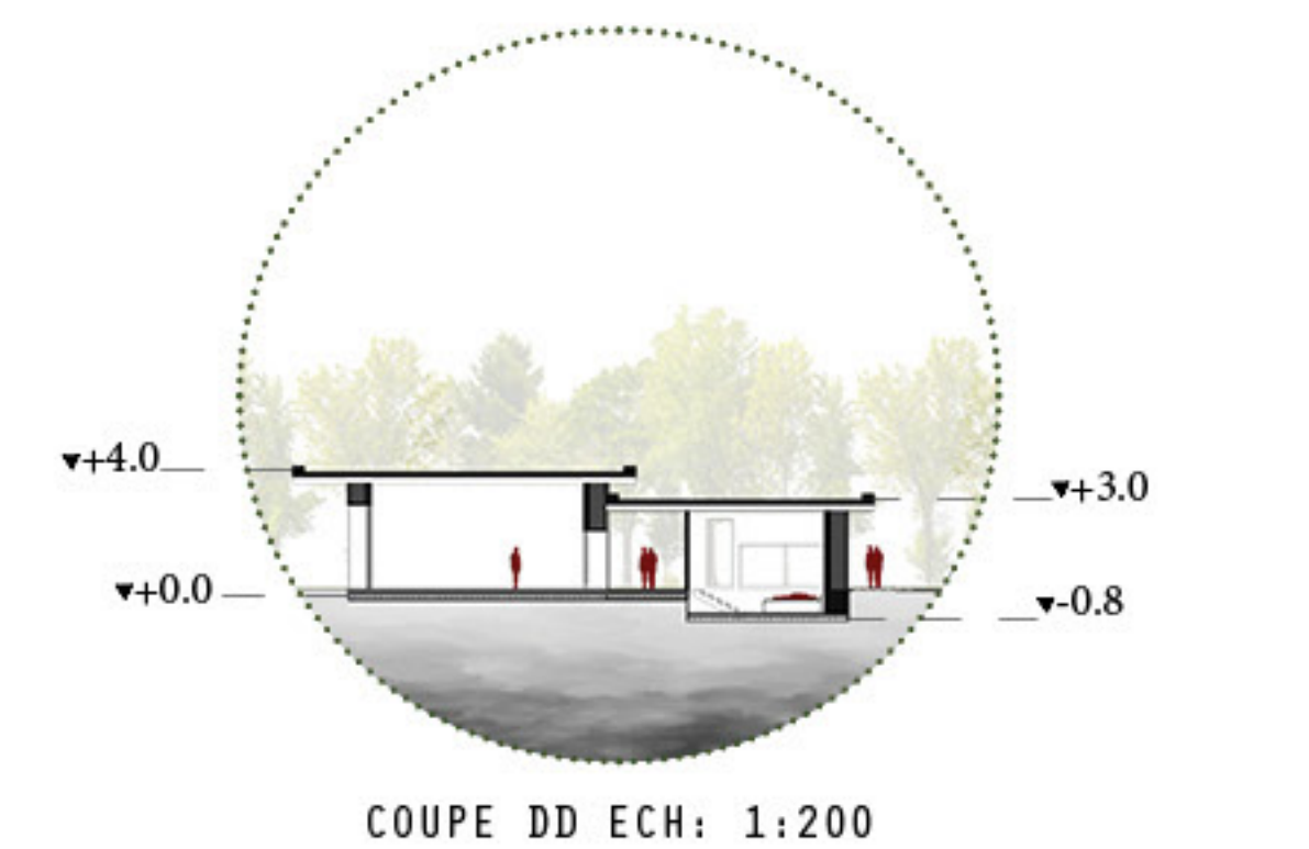
COUPE DD ECH: 1:200
