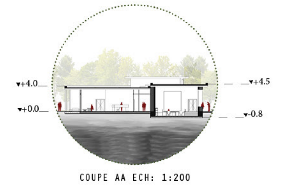
COUPE AA ECH: 1:200
