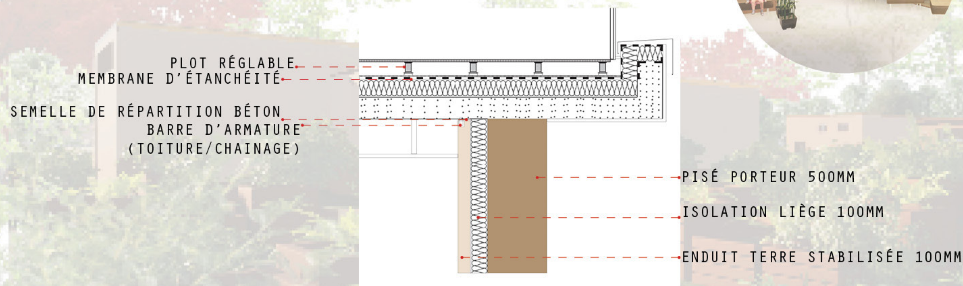
DÉTAIL COUPE DE TOITURE TERRASSE NON ACCESSIBLE
