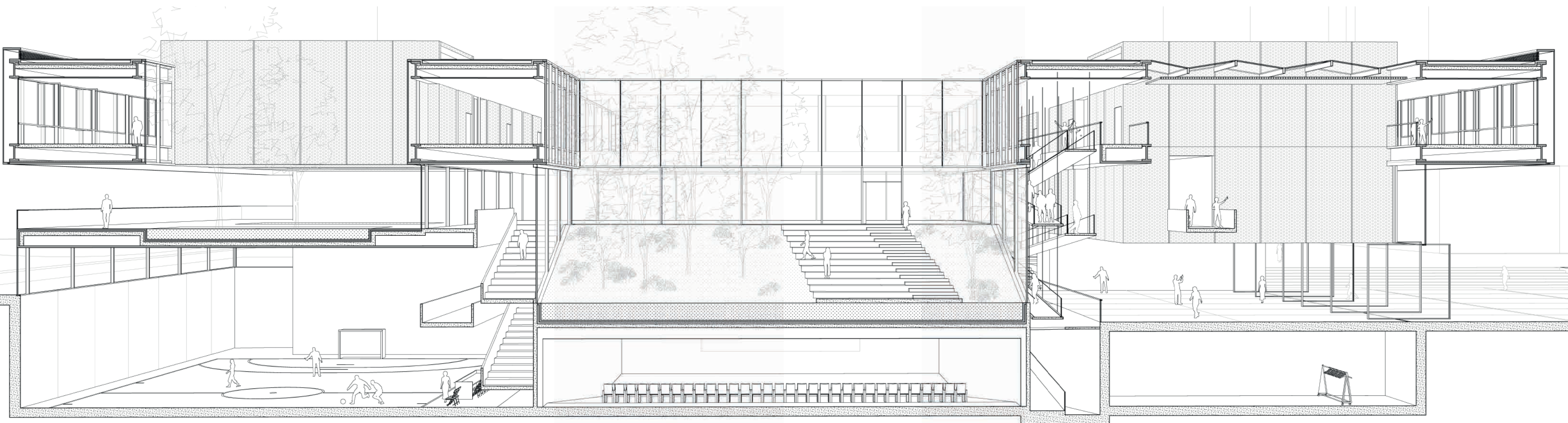
Coupe perspective dans le foyer de l'équipement
