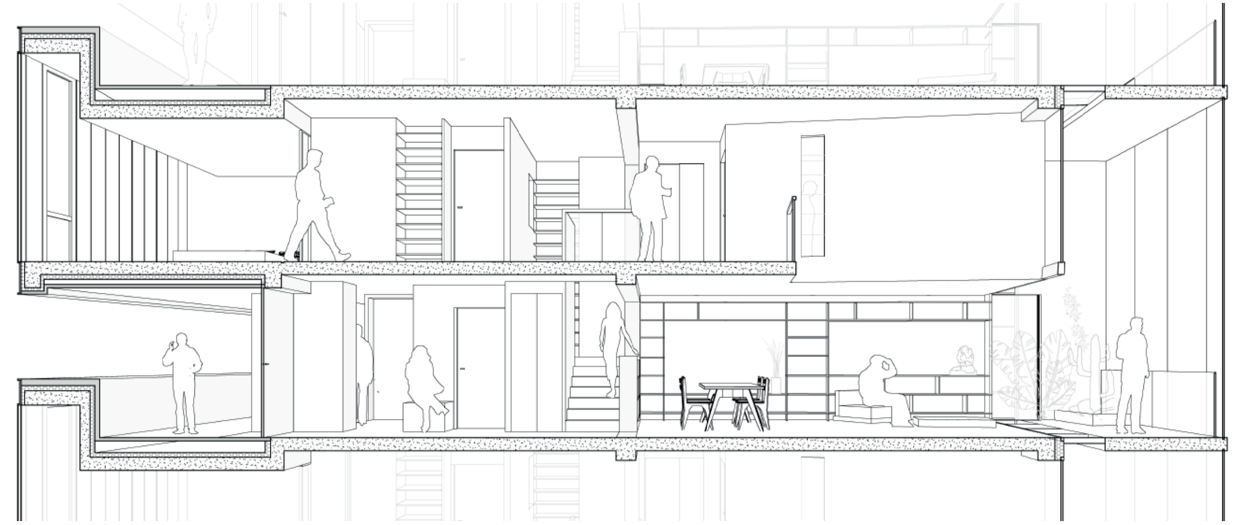
Coupe perspective d'un duplex type
