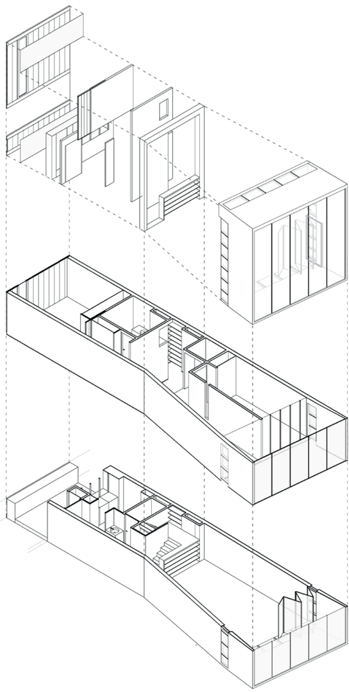
Axonométrie éclatée d'un duplex type succession de plans verticaux dans le logement
