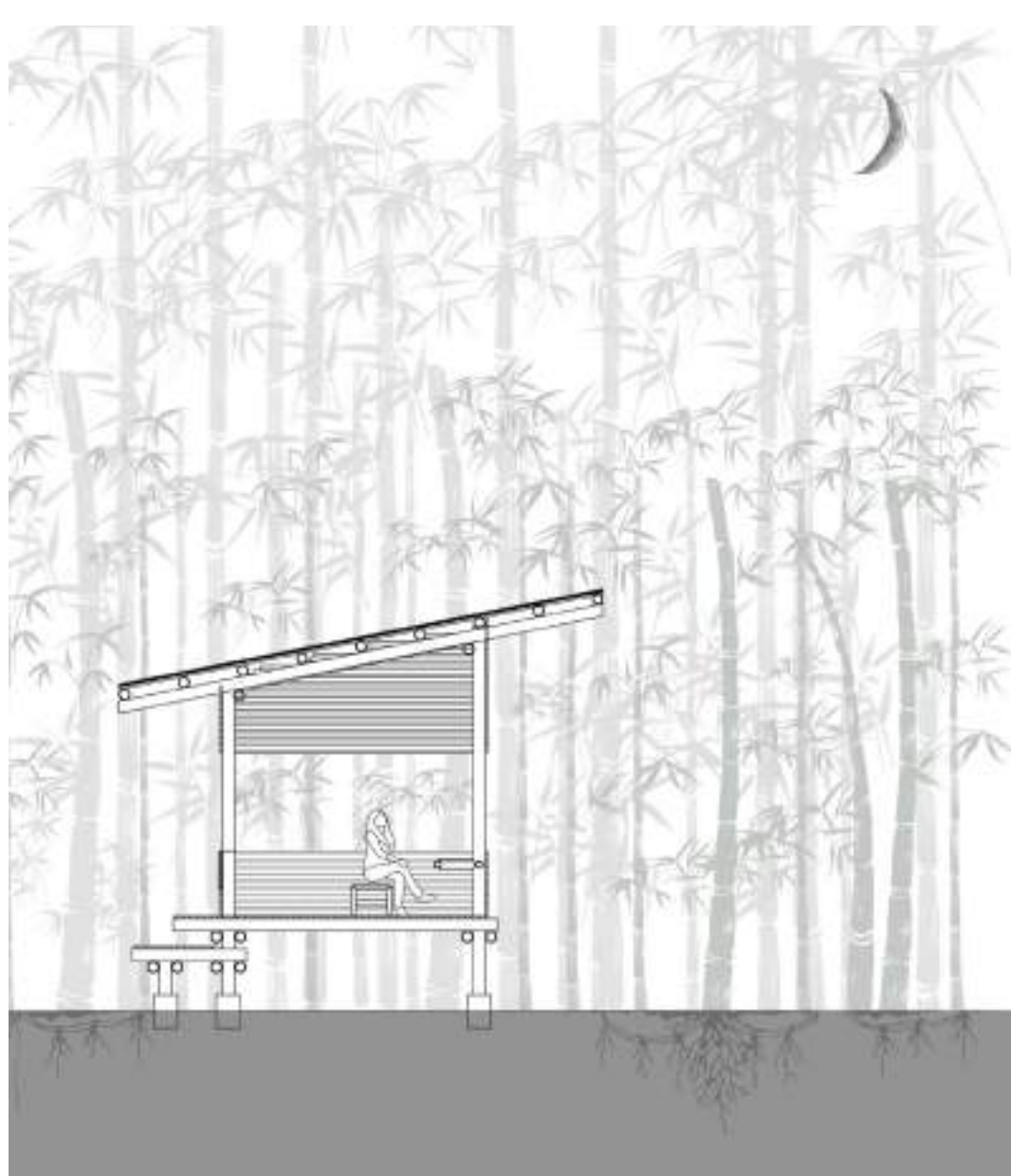
Coupe du pavillon de la clairière
