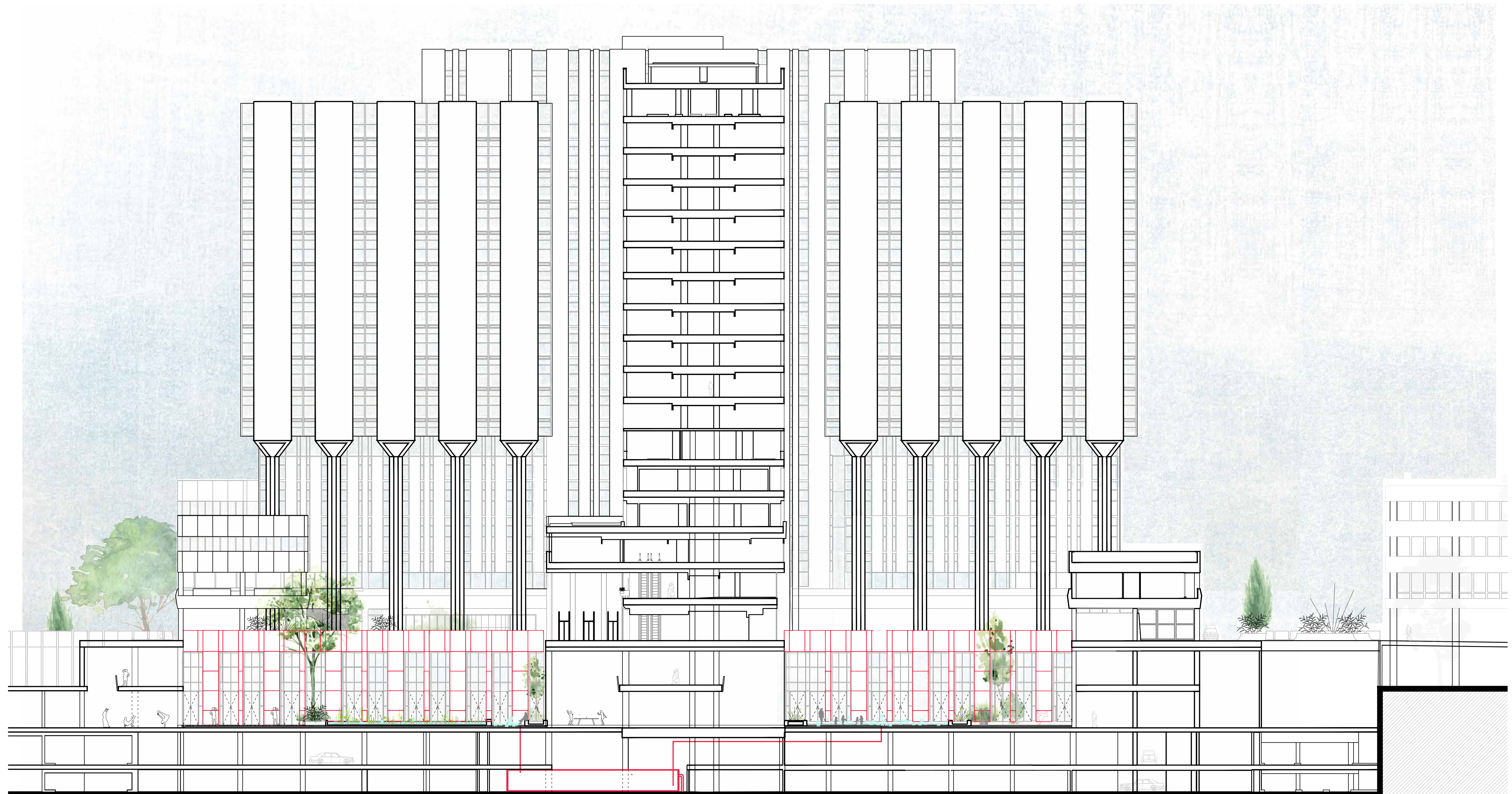
Coupe CC - 1/ 200 - Relation entre les façades existantes et projetées
