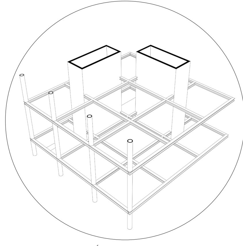
SCHEMA STRUCTUREL
