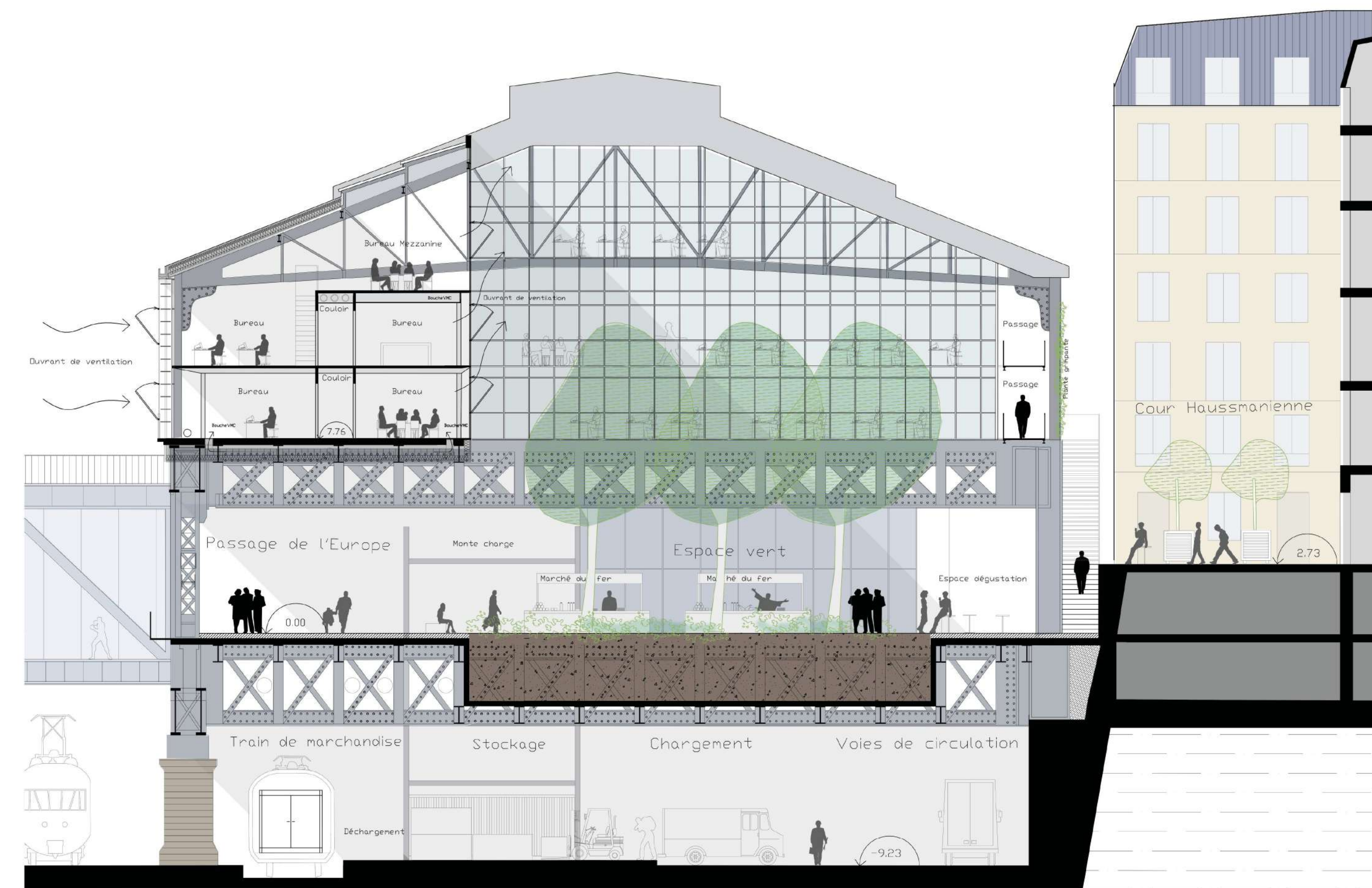
Coupe transversale dans un patio
