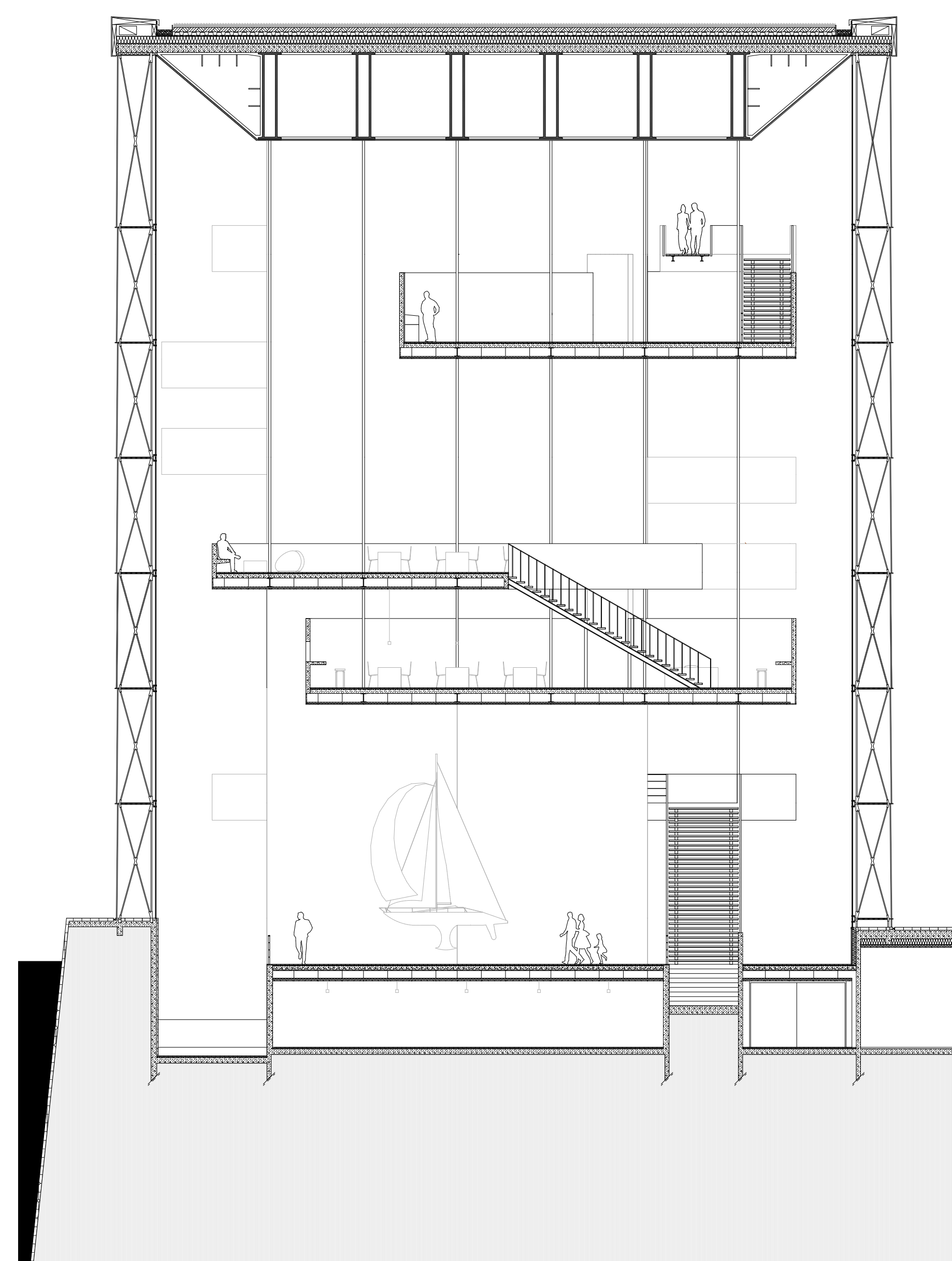
Coupe détail
