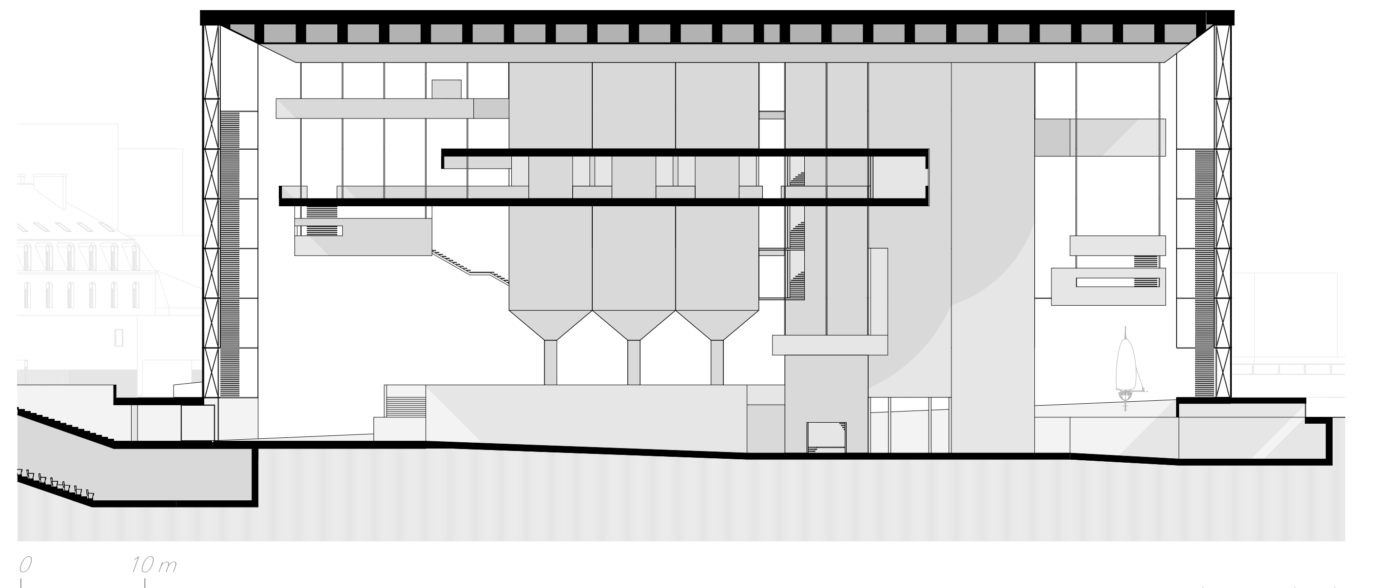
Coupe longitudinale
